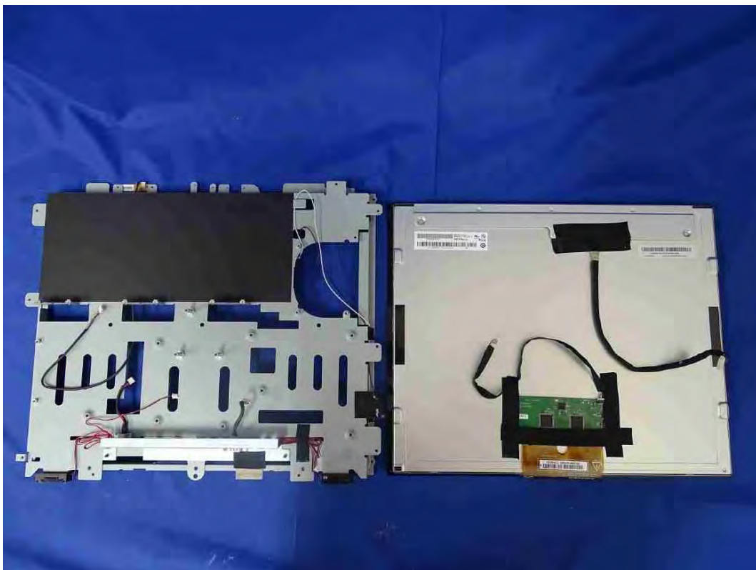
(49) EUT Photo
