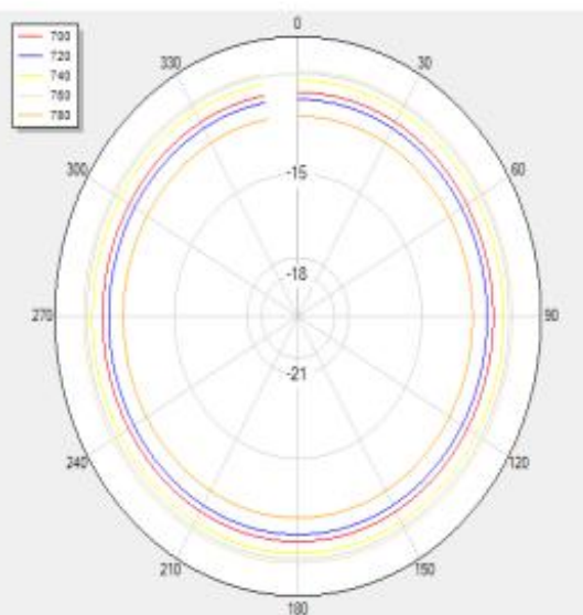
H Theta=0
