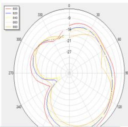
H Theta=90
