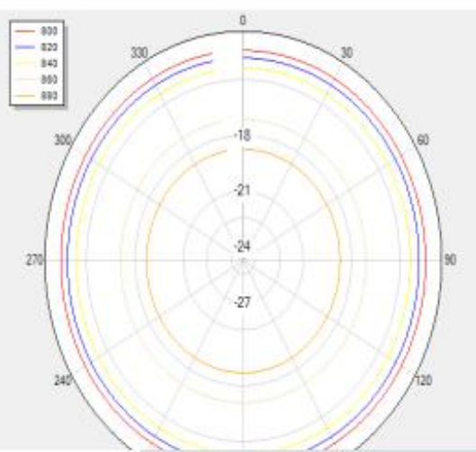
H Theta=0
