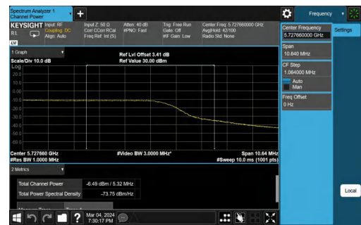
11N40MIMO-Ant1-5755-PASS
