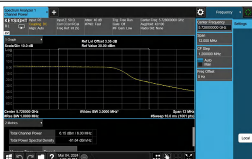
11AC20SISO-Ant0-5720_UNII-3-TPC_L-PASS
