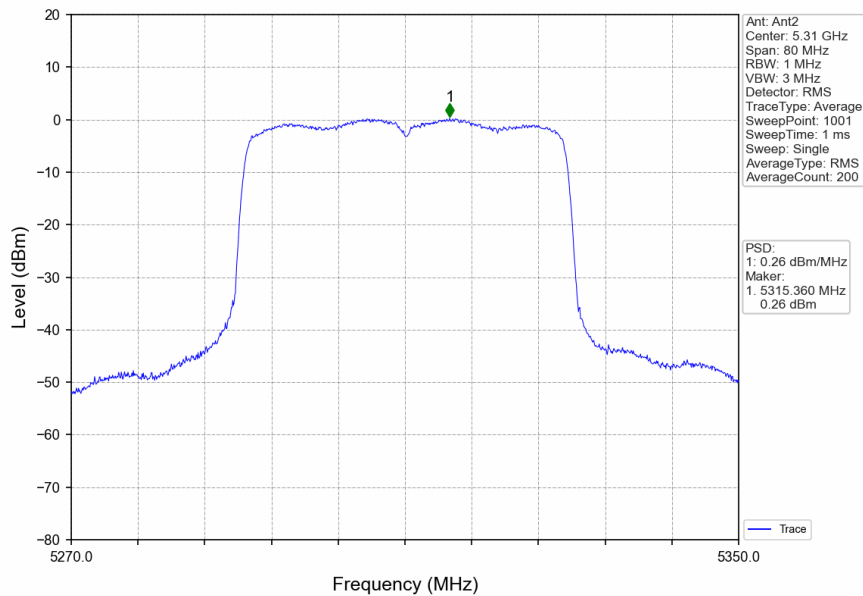
802.11ax(HEW40)_HCH_5310MHz_RU484_Left_Ant2_NTNV
