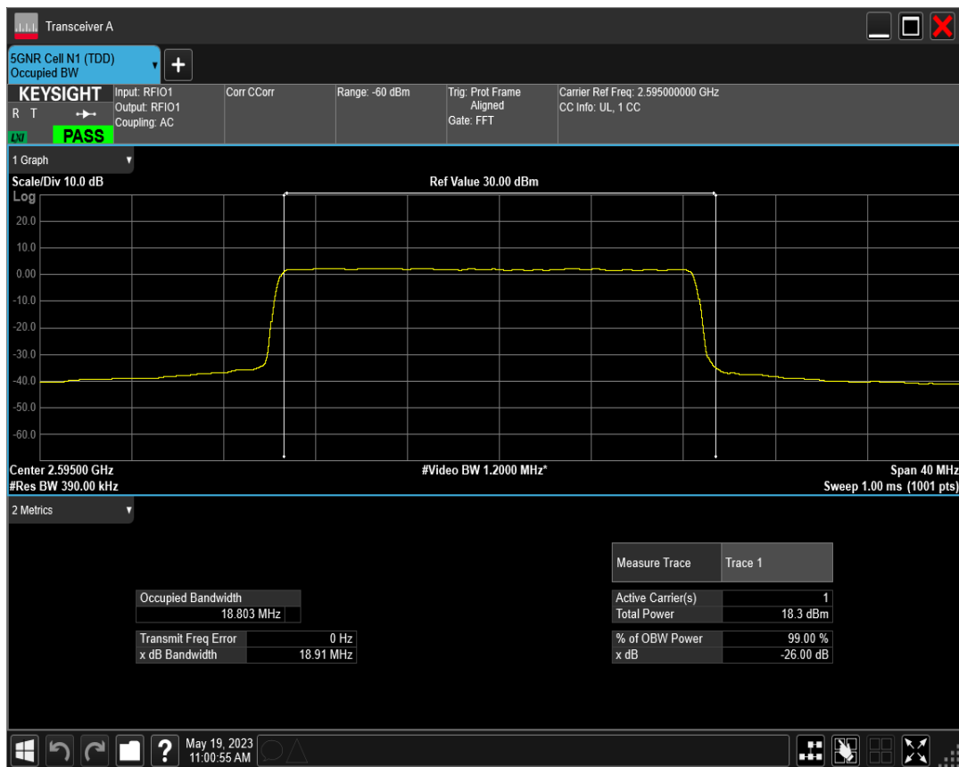
n38 SCS=15kHz CP_QPSK BW=20MHz Channel=519000 RB=106@0
