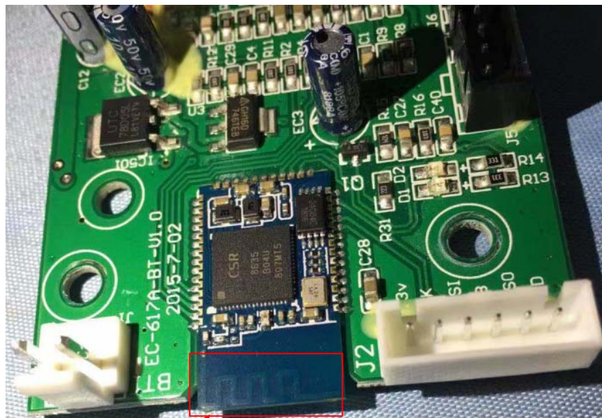
Antenna
