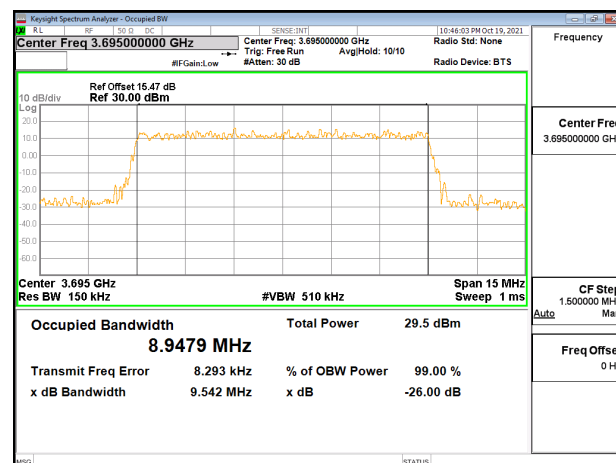
Band48_10MHz_QPSK_RB50_0_CH56690
