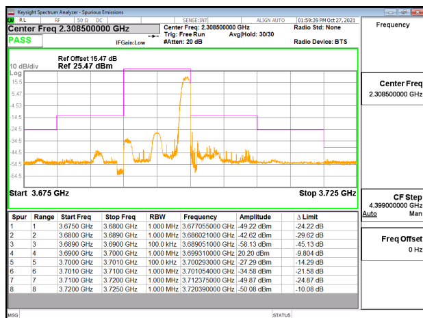
Emission Mask_Band48_10MHz_QPSK_RB1_49_CH56690
