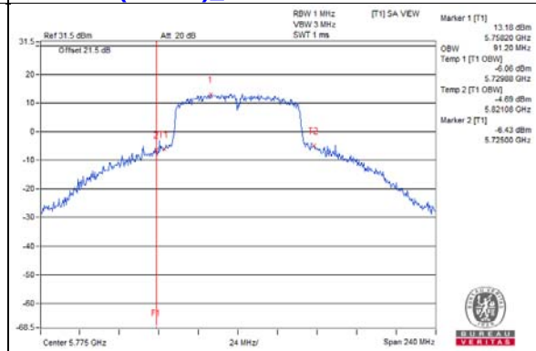
802.11ac (VHT80)_CH155
