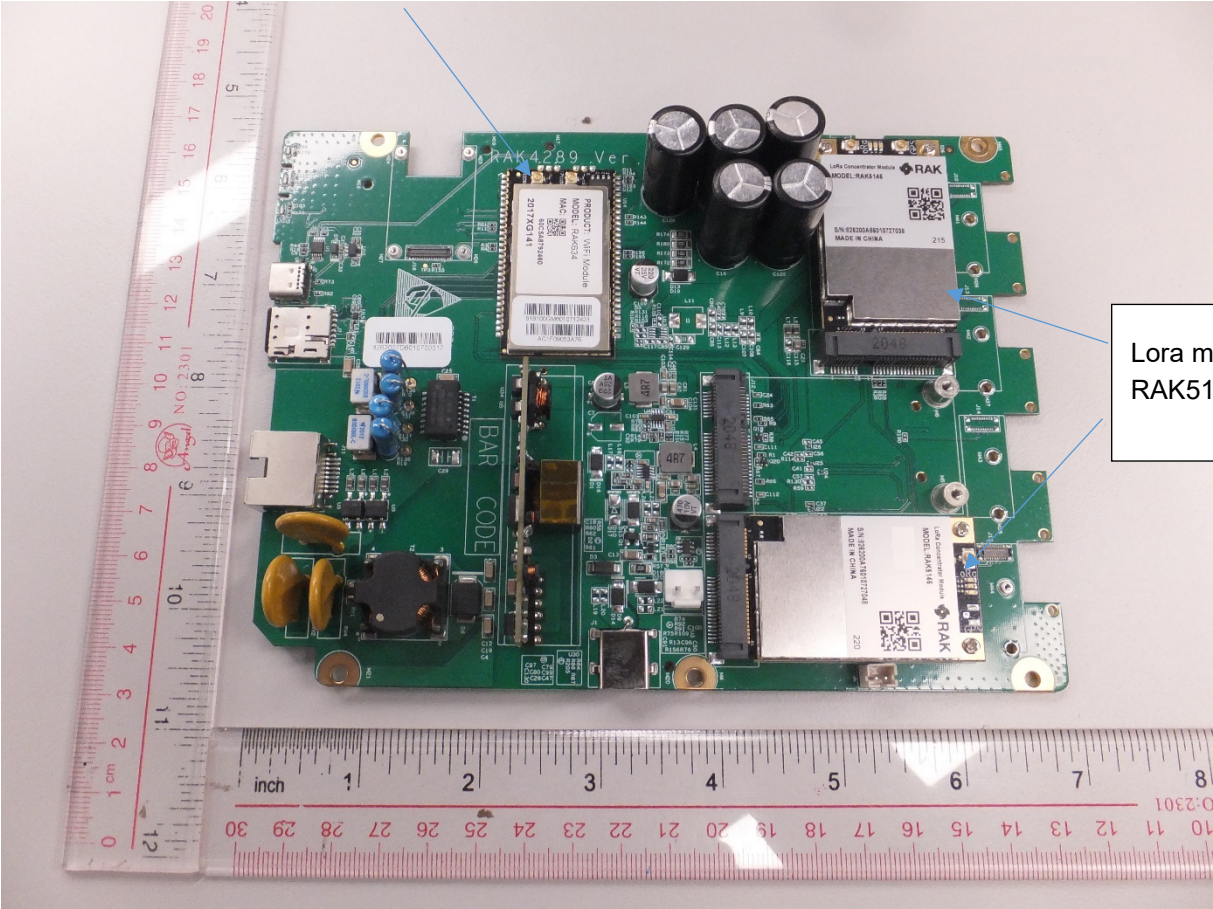
WIFI module RAK634
