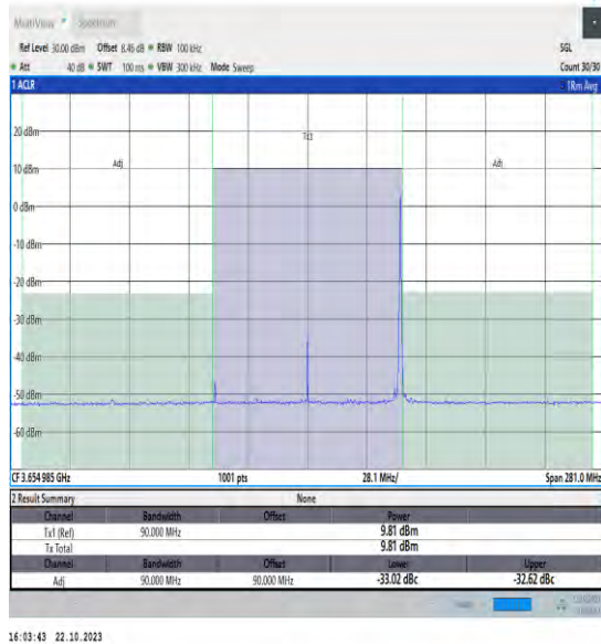
NTNV_N48_PC3_30_90_H_TID18_#1_-90_90
