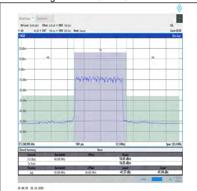
NTNV_N48_PC3_30_40_L_TID1_#1_-40_40
