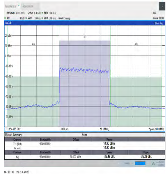
NTNV_N48_PC3_30_90_H_TID1_#1_-90_90
