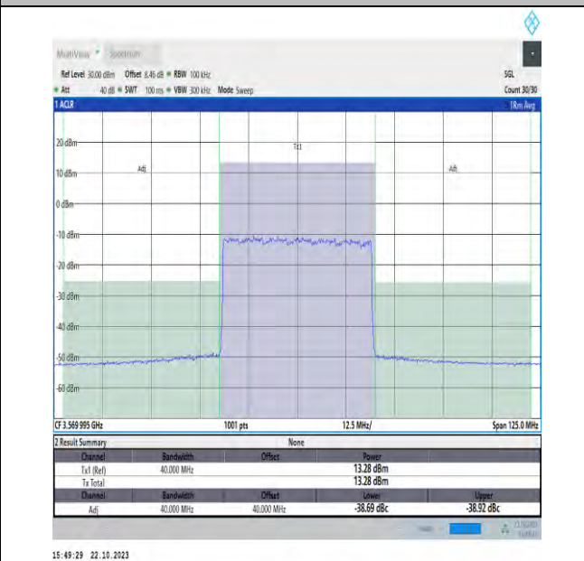
NTNV_N48_PC3_30_40_L_TID16_#1_-40_40
