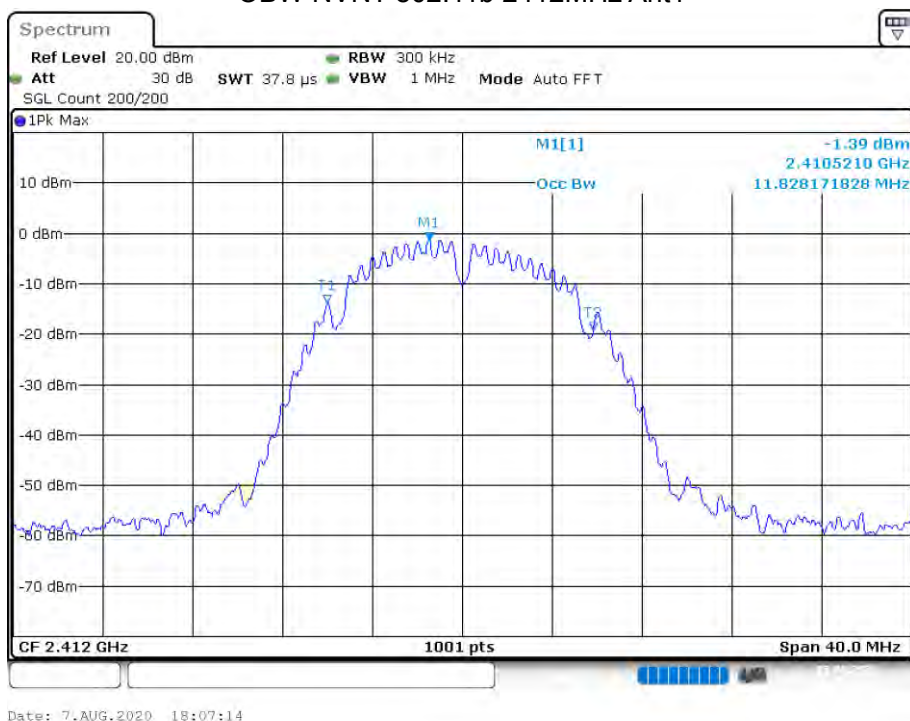
OBW NVNT 802.11b 2412MHz Ant1
