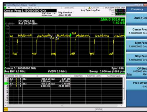
802.11ac(40MHz) 5190MHz
