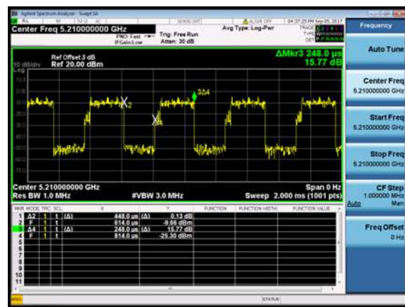
802.11ac(80MHz) 5210MHz
