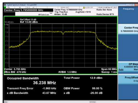
Channel 159(5795MHz)
