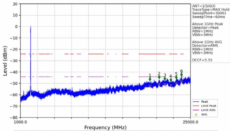
802.11ax(HEW40) MCH 2437MHz_RU484_Left_Ant1 (SISO) NTNv
