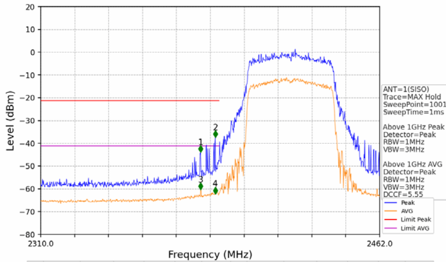
802.11ax(HEW40) LCH 2422MHz_RU484_Left_Ant1 (SISO) NTNv
