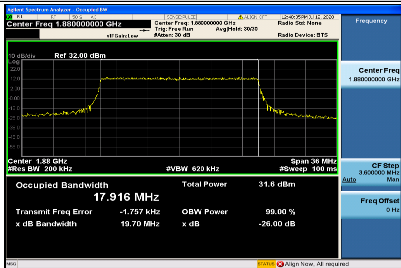
Band2-20MHz-QPSK-18900-100RB#0-17.916
