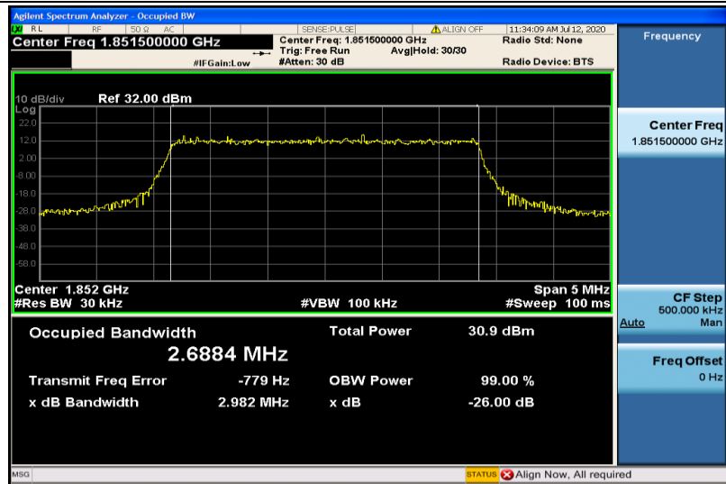
Band2-3MHz-QPSK-18615-15RB#0-2.6884
