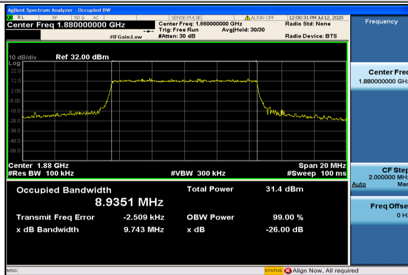
Band2-10MHz-QPSK-18900-50RB#0-8.9351
