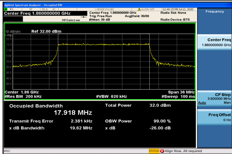
Band2-20MHz-QPSK-18700-100RB#0-17.918
