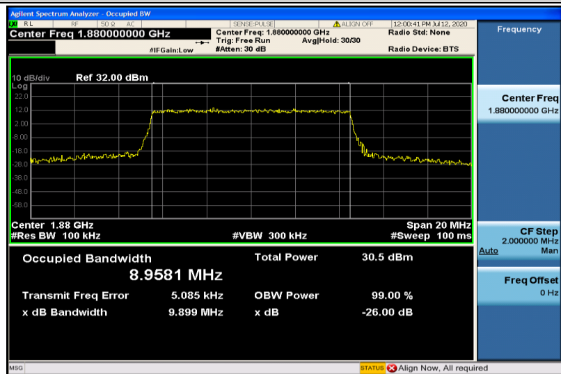
Band2-10MHz-16QAM-18900-50RB#0-8.9581
