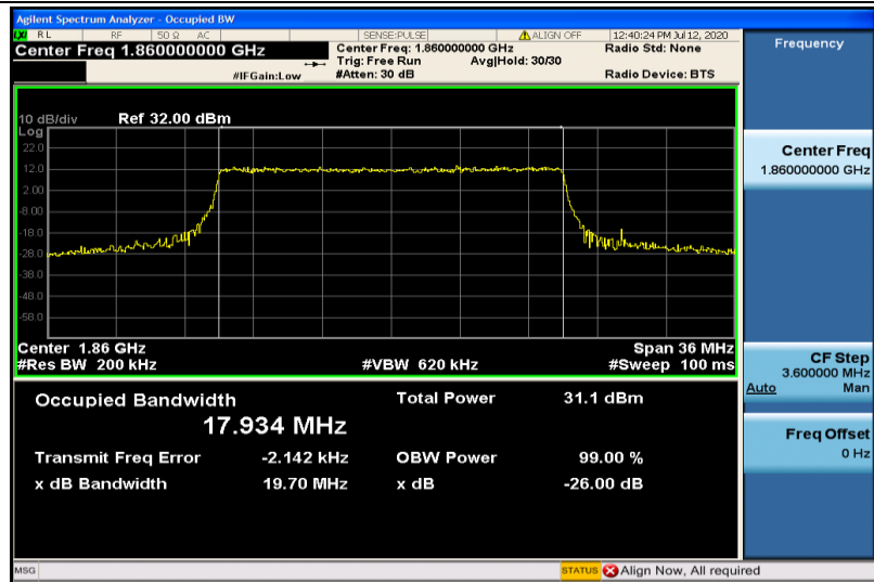
Band2-20MHz-16QAM-18700-100RB#0-17.934
