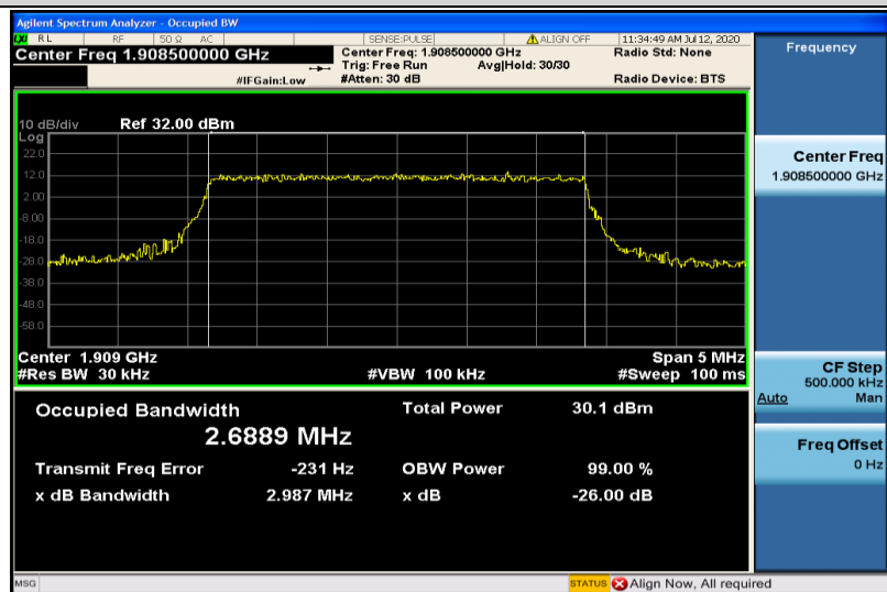
Band2-3MHz-QPSK-19185-15RB#0-2.6889
