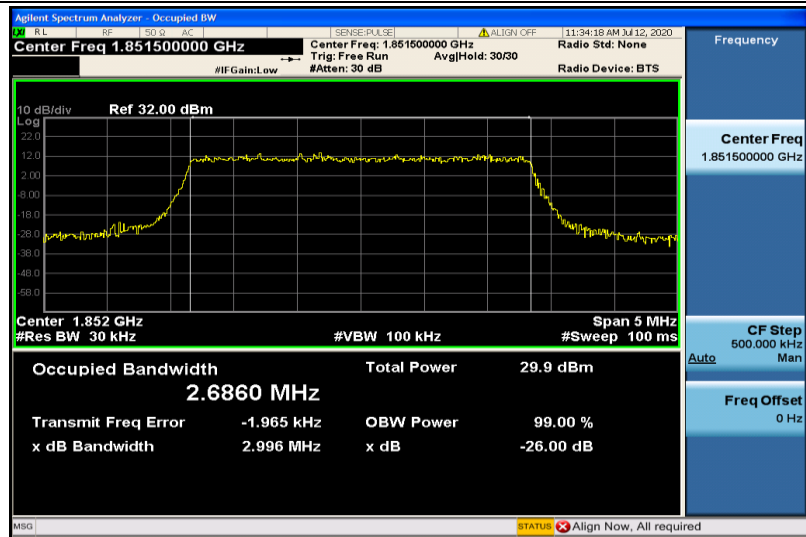
Band2-3MHz-16QAM-18615-15RB#0-2.6860
