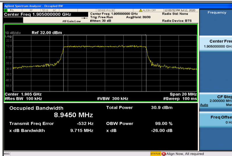
Band2-10MHz-QPSK-19150-50RB#0-8.9450
