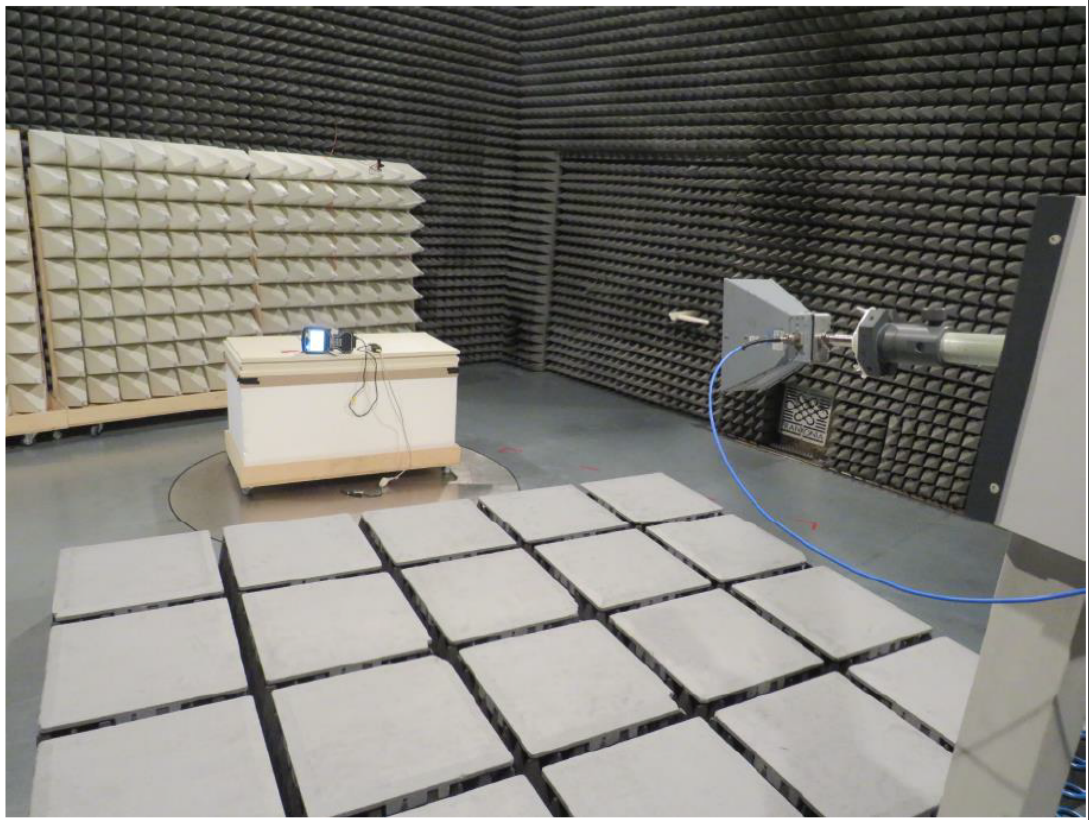
Test setup 1000-13000MHz
