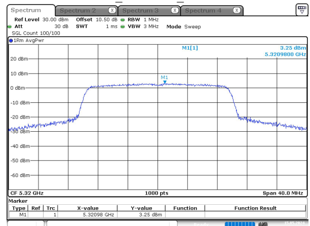
ax20_5320MHz_Chain 0
