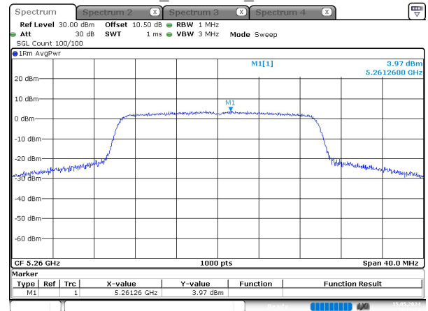
ax20_5260MHz_Chain 0
