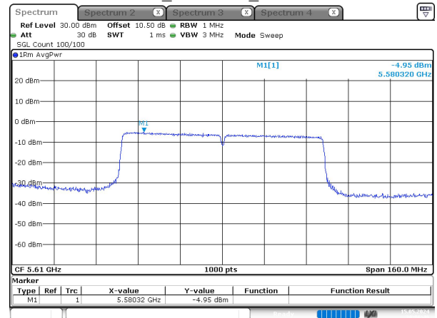
ac80_5610MHz_Chain 0
