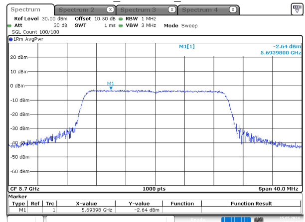
ax20_5700MHz_Chain 0
