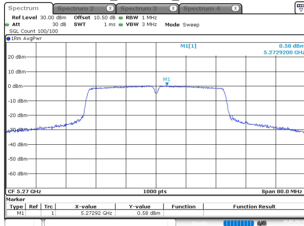
n40_5270MHz_Chain 0
