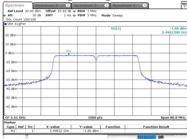
n40_5510MHz_Chain 0
