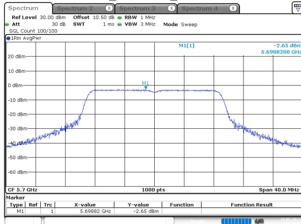
n20_5700MHz_Chain 0
