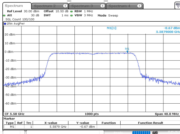
ax20_5580MHz_Chain 0
