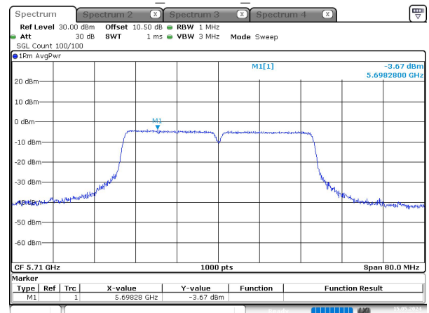
n40_5710MHz_Chain 0
