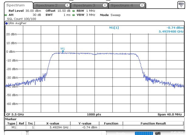
ax20_5500MHz_Chain 0
