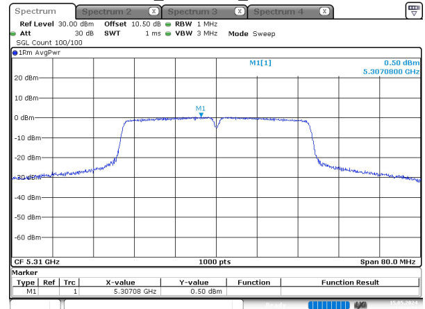
n40_5310MHz_Chain 0
