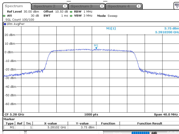
ax20_5280MHz_Chain 0
