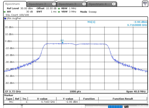
n20_5720MHz_Chain 0
