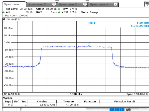
ac80_5530MHz_Chain 0
