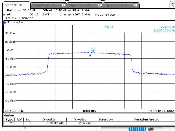
ac80_5290MHz_Chain 0
