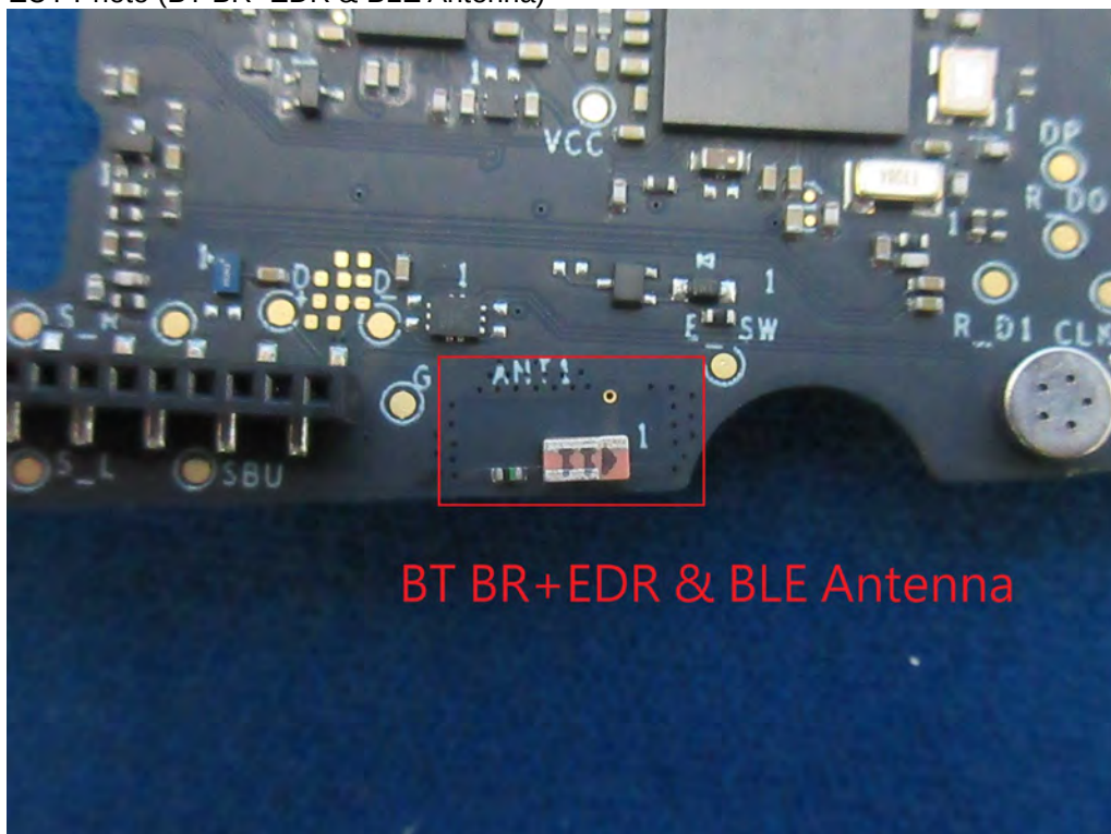
(6) EUT Photo (BT BR+EDR & BLE Antenna)
