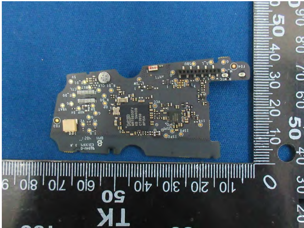
(6) EUT Photo (BT BR+EDR & BLE Antenna)
