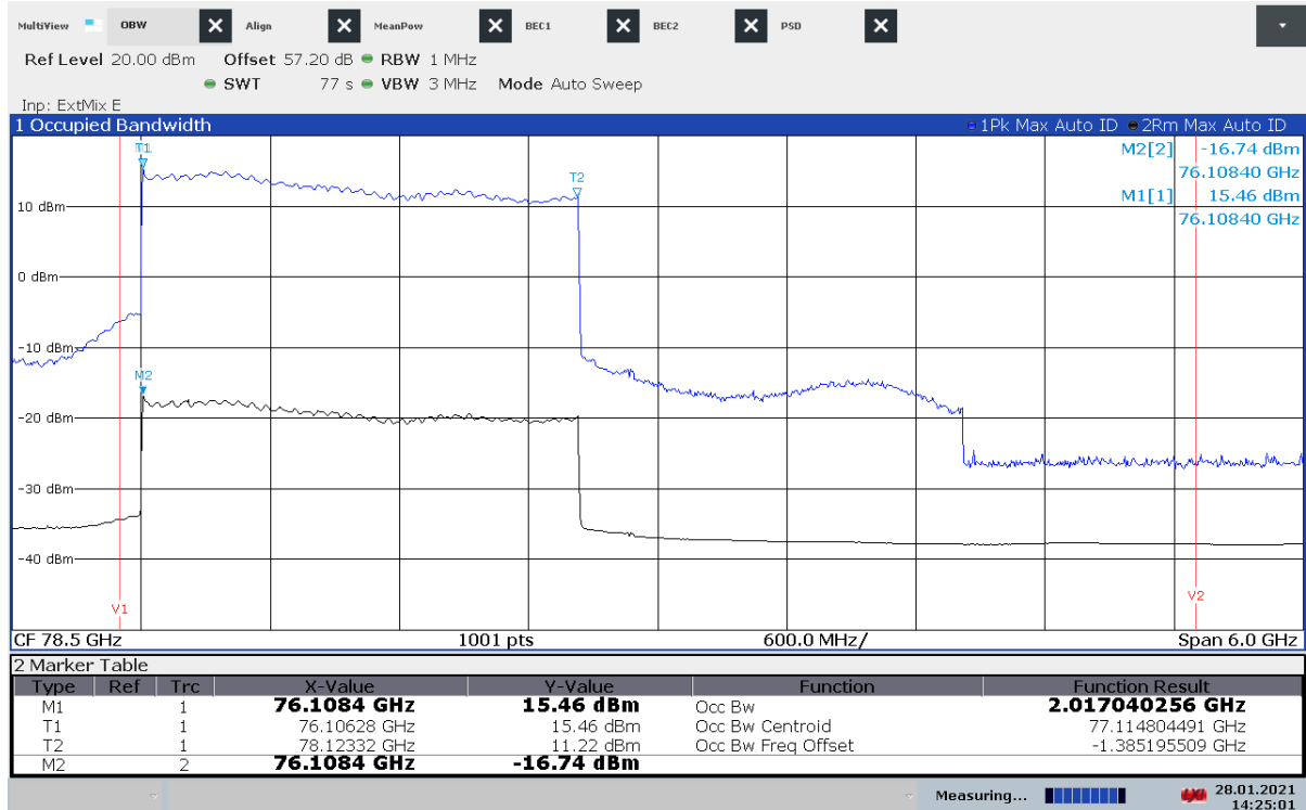
Plot 53: OBW, -10 °C / V nom , Mode 5
