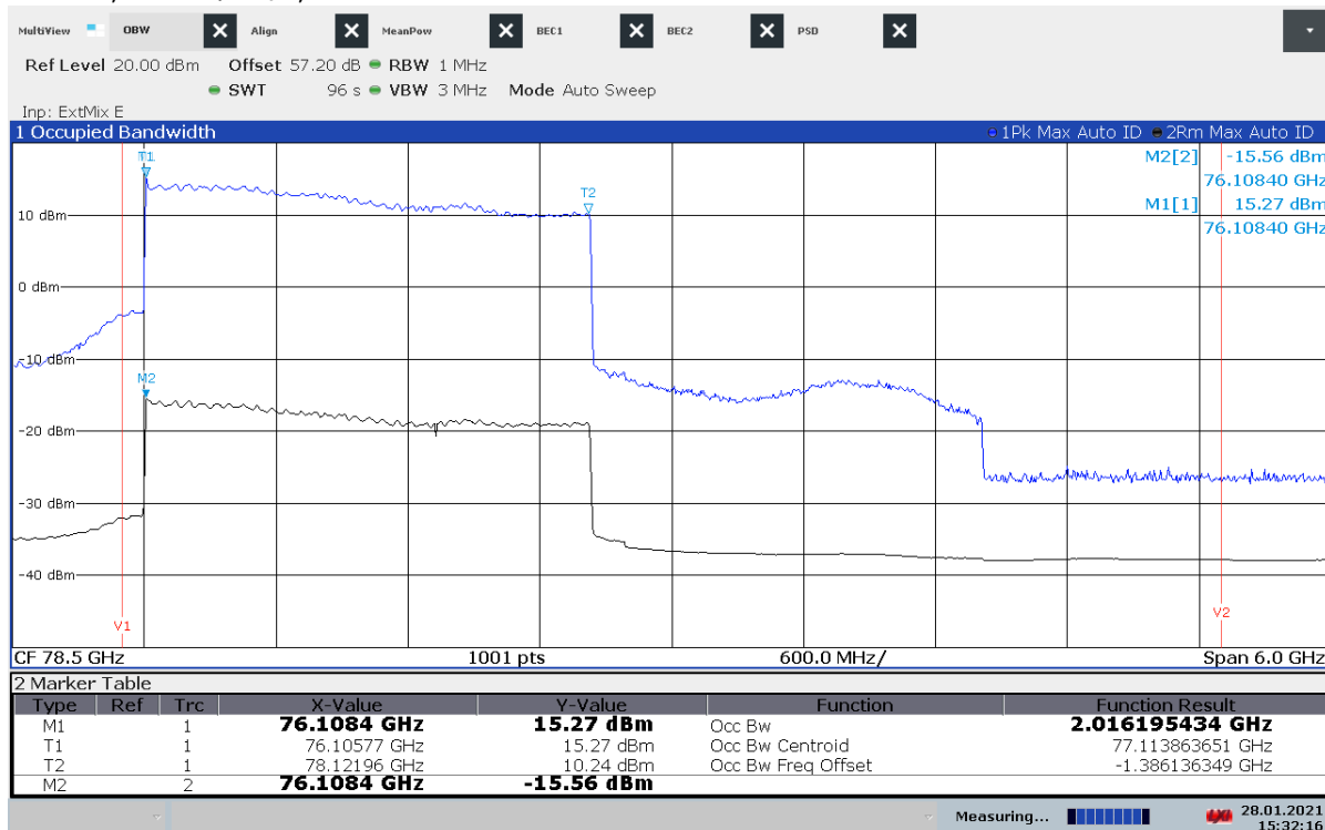
Plot 66: OBW, +30 °C / V nom , Mode 6
