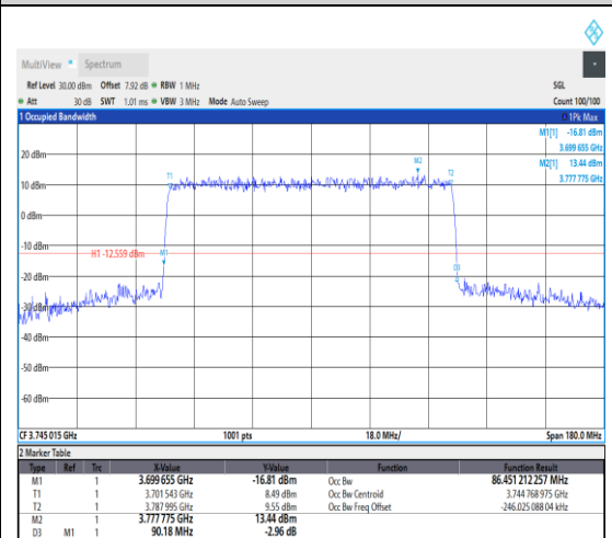
1-N77-3700-3980--30-90-L-4-DFT-64QAM-O
