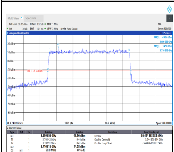
1-N77-3700-3980--30-90-L-3-DFT-16QAM-O
