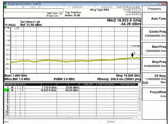
CSE B4 3M CH19965 QPSK(1,14) 1G-18G
