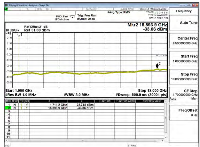
CSE B4 1.4M CH19957 16QAM(1,2) 1G-18G
