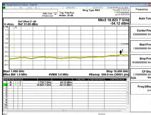
CSE B4 3M CH20175 QPSK(1,7) 1G-18G
