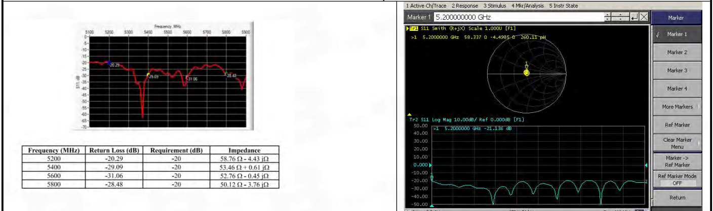
5000MHz Dipole
