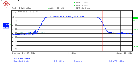
802.11n(HT20)
