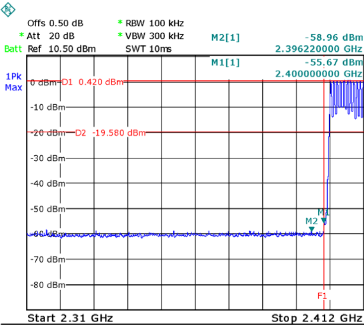
GFSK Band edge Hopping-left side
