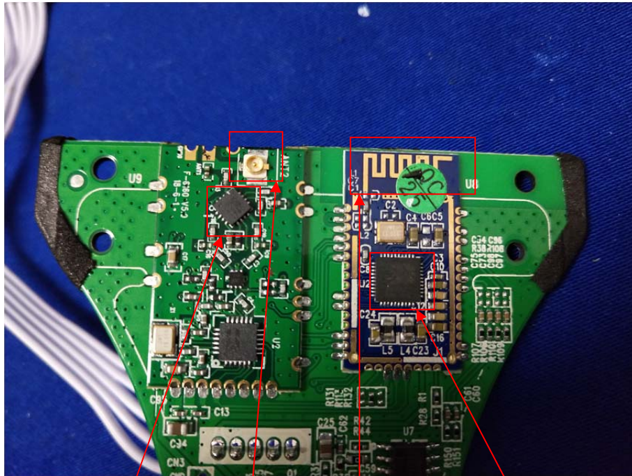
5.8G module 5.8G antenna BT antenna BT module
