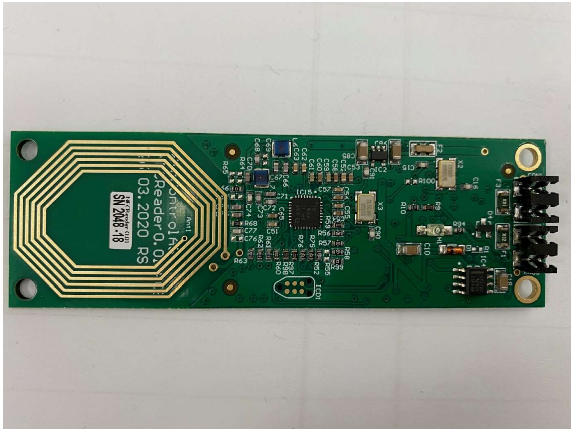
NFC_Reader0.01.PCB TOP
