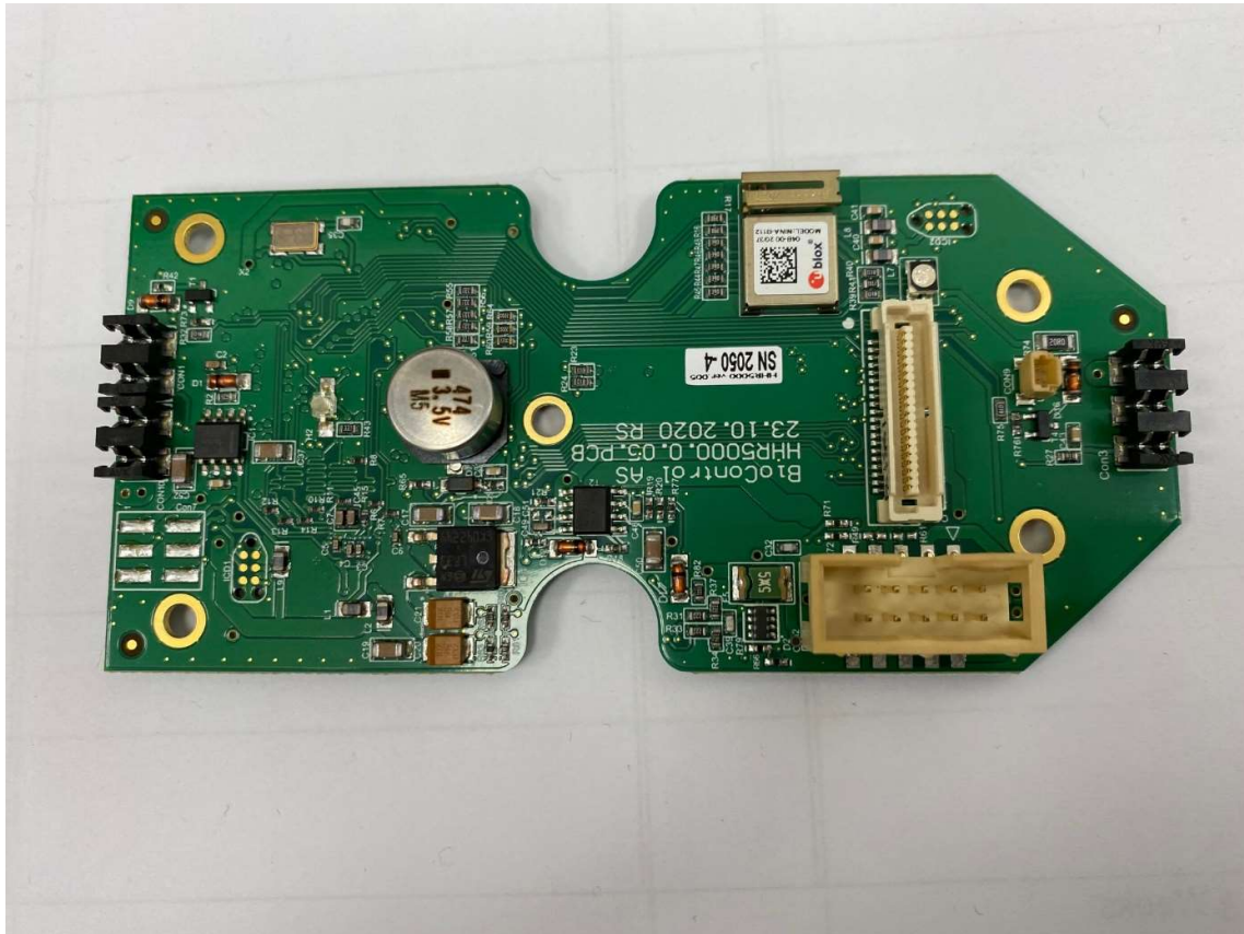
HHR5000.0.05.PCB TOP
