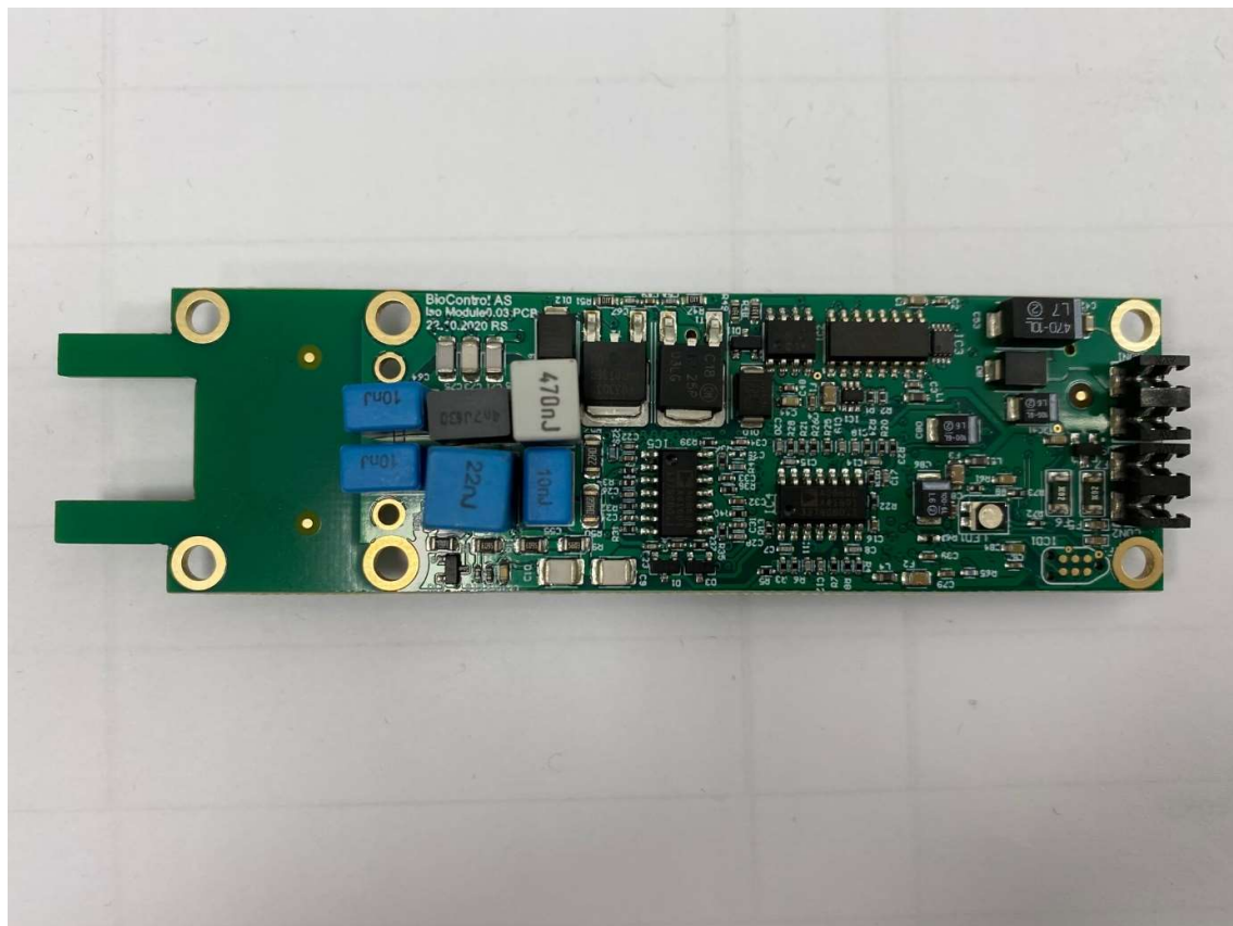
ISO_Module0.03.PCB TOP
