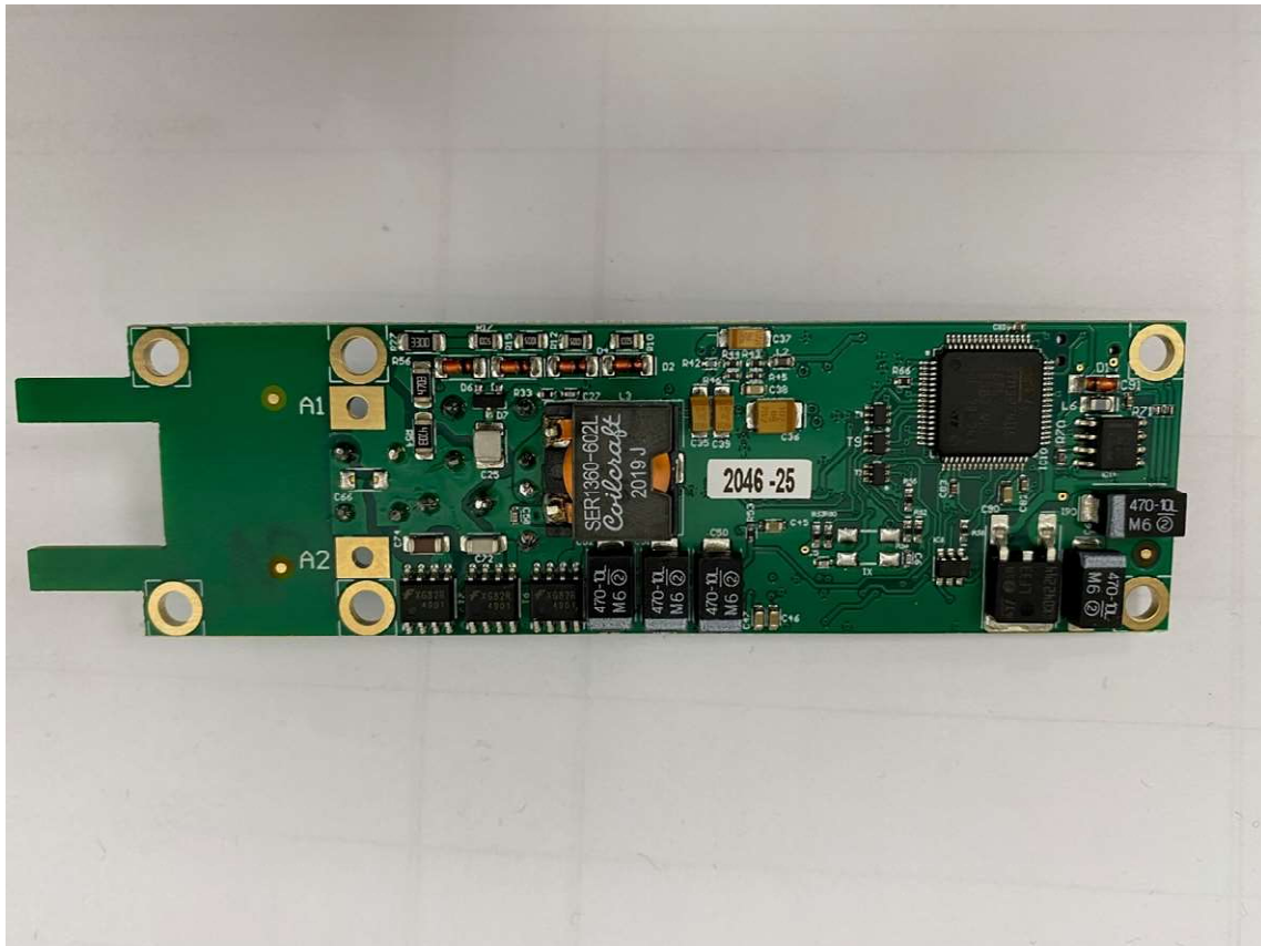
ISO_Module0.03.PCB BOTTOM
