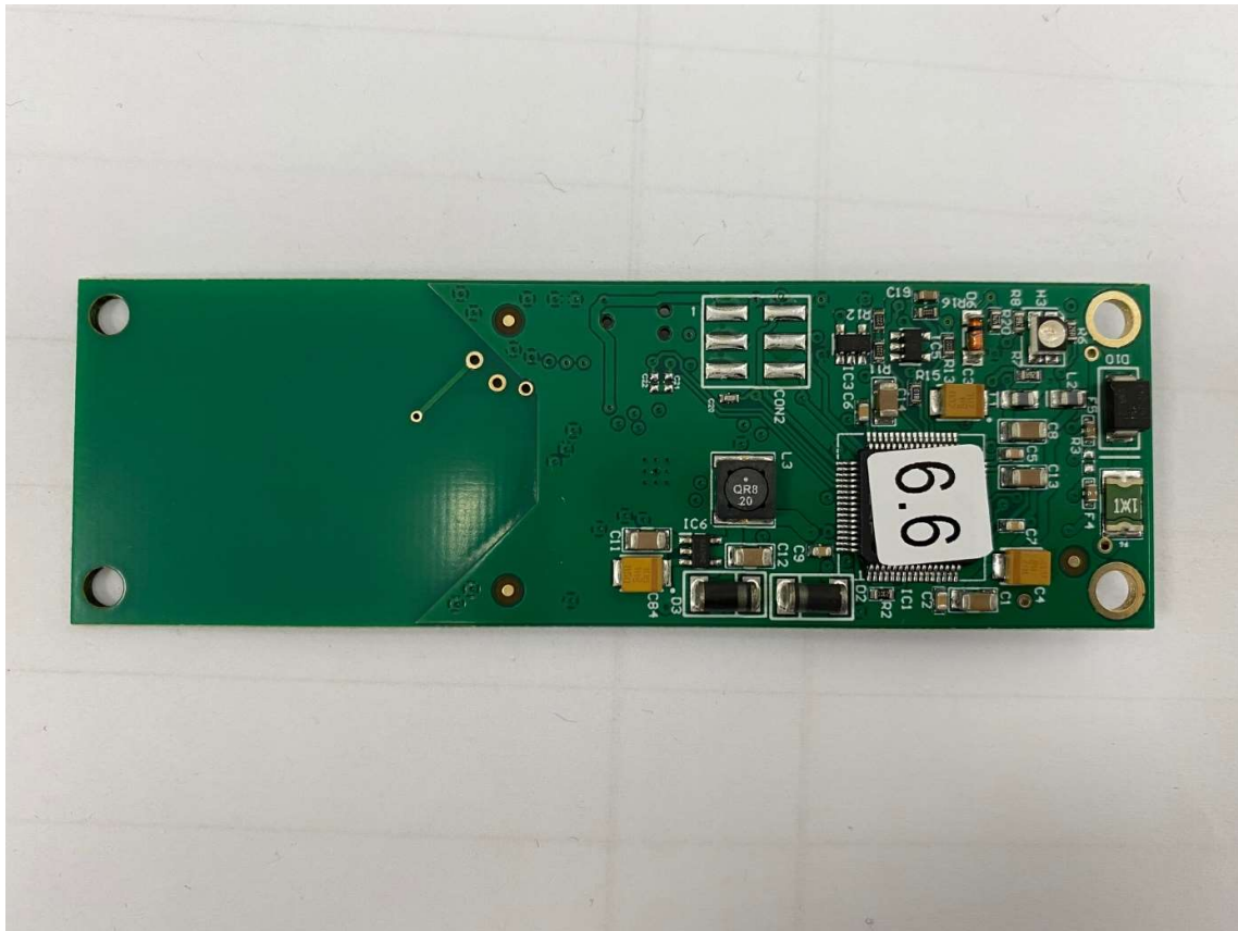
NFC_Reader0.01.PCB BOTTOM
