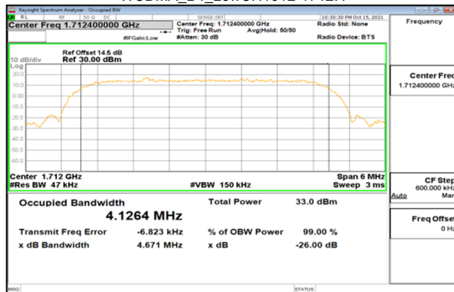
WCDMA_B4_LowCH1312-1712.4
