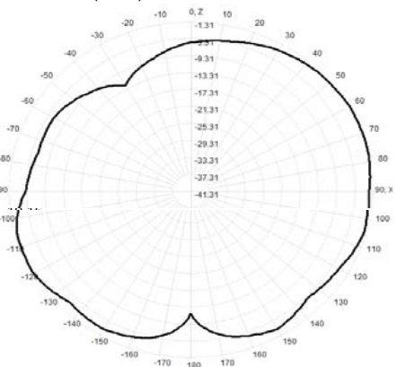
900.0MHz Total(E1-XZ), Max= -1.31dBi
