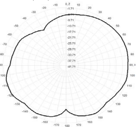
910.0MHz Total(E1-XZ), Max= -1.71dBi
