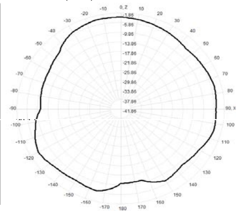
930.0MHz Total(E1-XZ), Max= -3.57dBi
