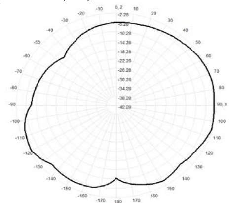
920.0MHz Total(E1-XZ), Max= -2.57dBi
