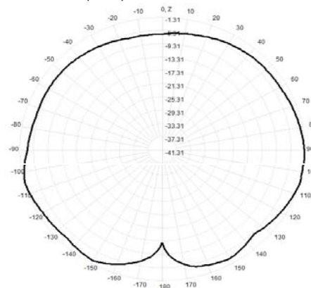
900.0MHz Total(E2-YZ), Max= -1.40dBi
