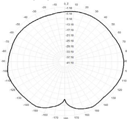
860.0MHz Total(E2-YZ), Max= -1.30dBi
