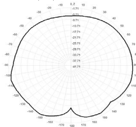
910.0MHz Total(E2-YZ), Max= -1.84dBi
