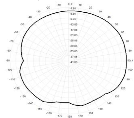
930.0MHz Total(E2-YZ), Max= -1.86dBi
