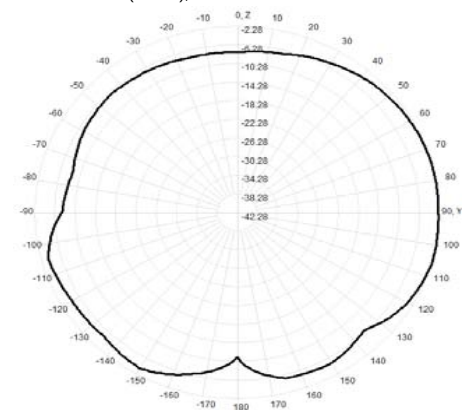
920.0MHz Total(E2-YZ), Max= -2.42dBi
