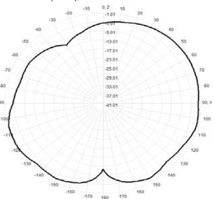
890.0MHz Total(E1-XZ), Max= -1.20dBi
