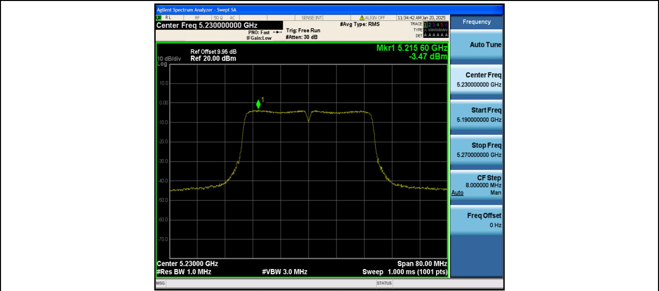
11AC40MIMO_Ant2_5230
