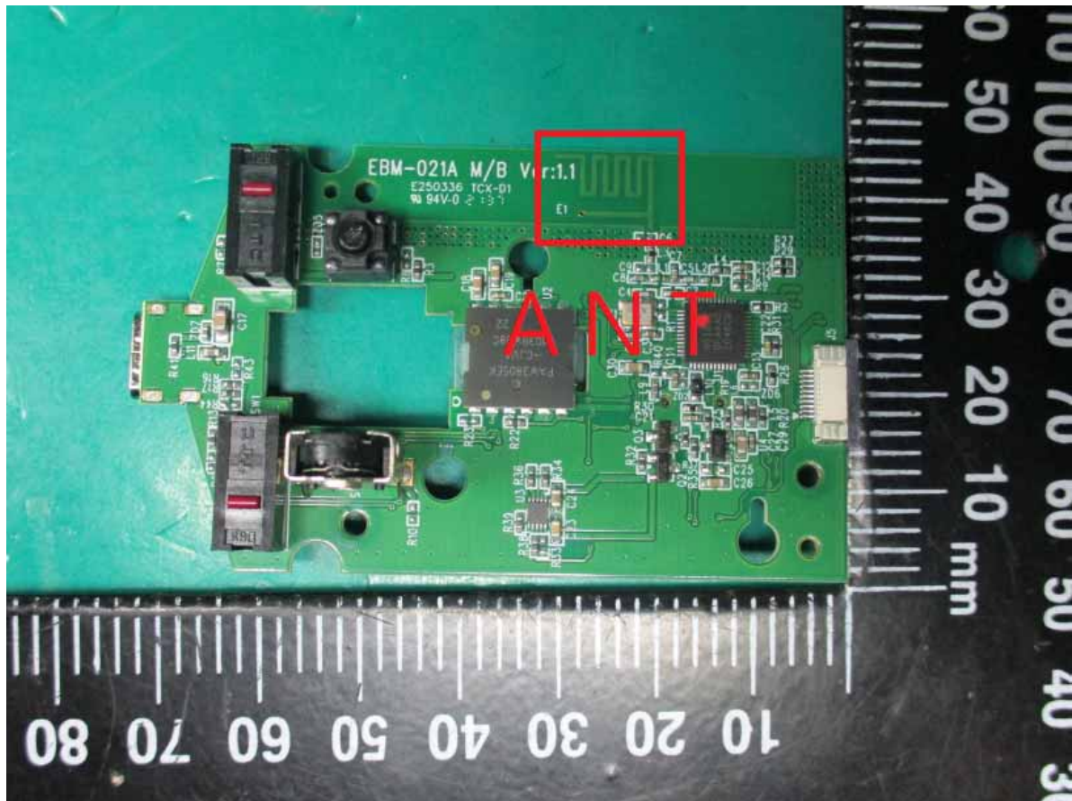
Antenna
