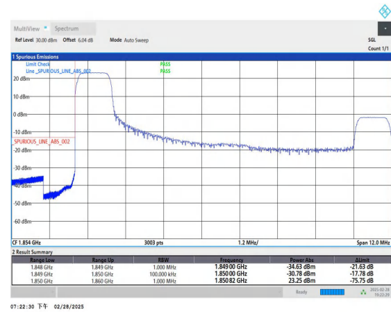
Band2_10MHz_QPSK_18650_1RB#0
