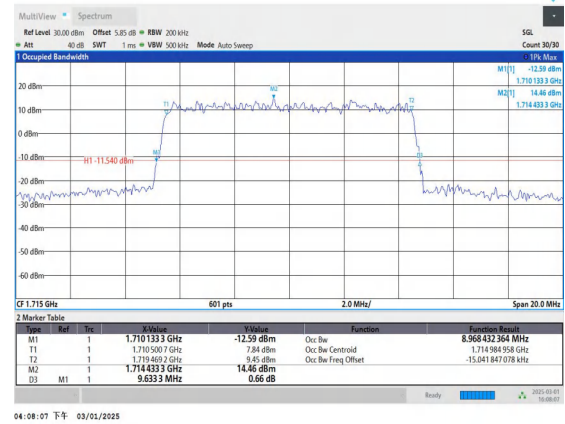
Band4-10MHz-QPSK-20000-50RB#0-PASS
