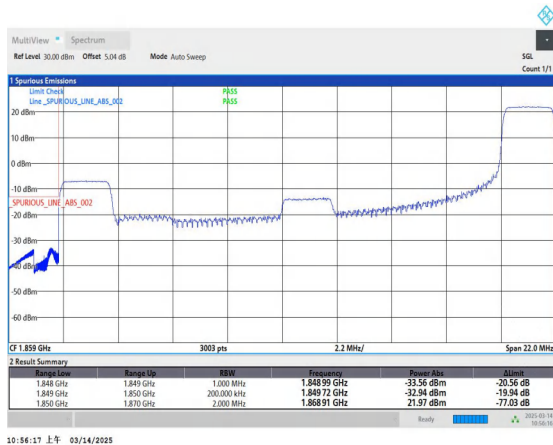
Band2_20MHz_QPSK_18700_1RB#99
