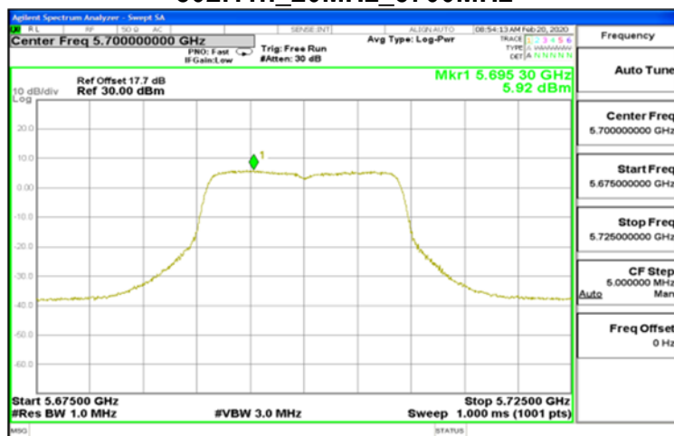
802.11n_20MHz_5700MHz
