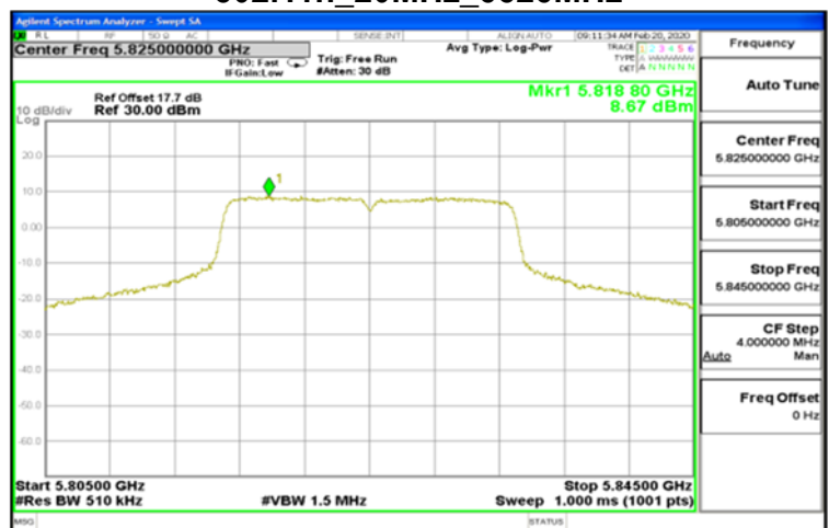
802.11n_20MHz_5825MHz
