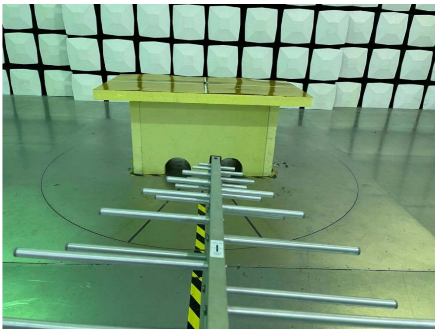
Below 1GHz(BLE)
