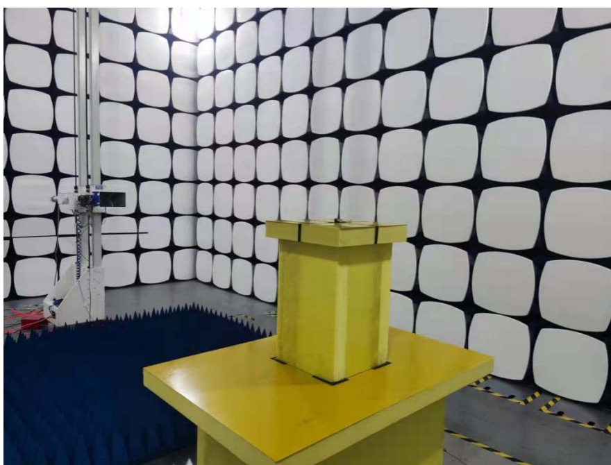
Above 1GHz(BLE)
