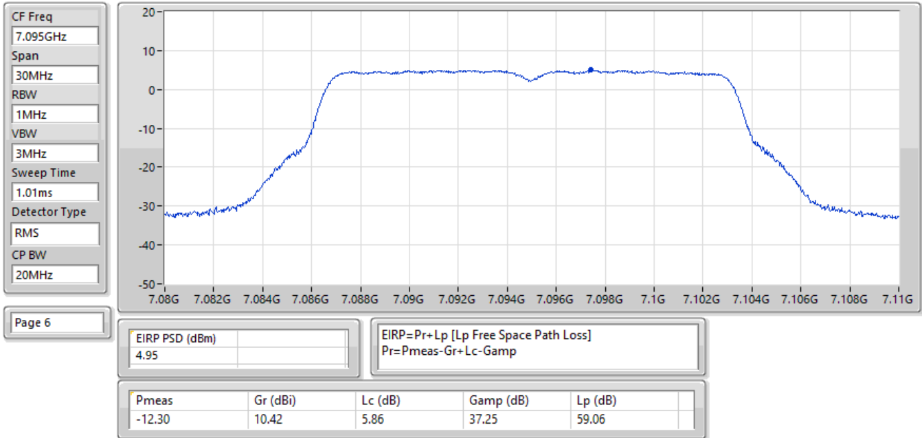
EIRP PSD;Band:7.0G;a20;BWch:20MHz;Nss:1,(6D);Nant:1;Ch:7095MHz;TX
