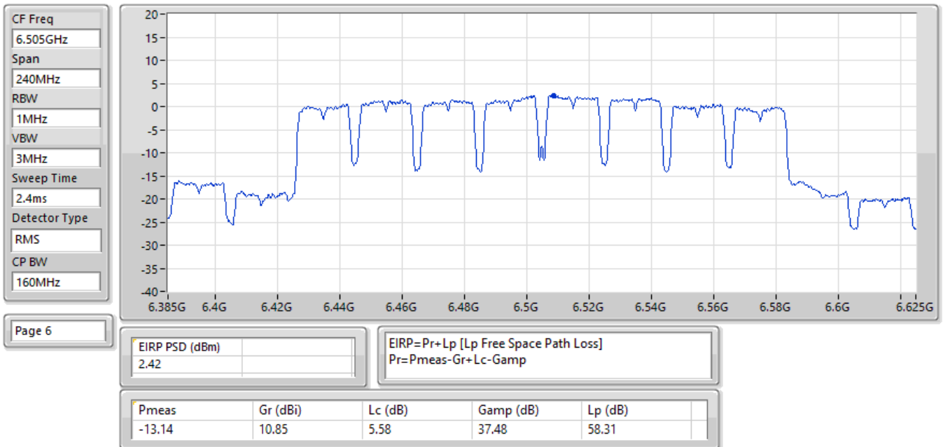
EIRP PSD;Band:6.4G;a160;BWch:160MHz;Nss:1,(6D);Nant:1;Ch:6505MHz;TX
