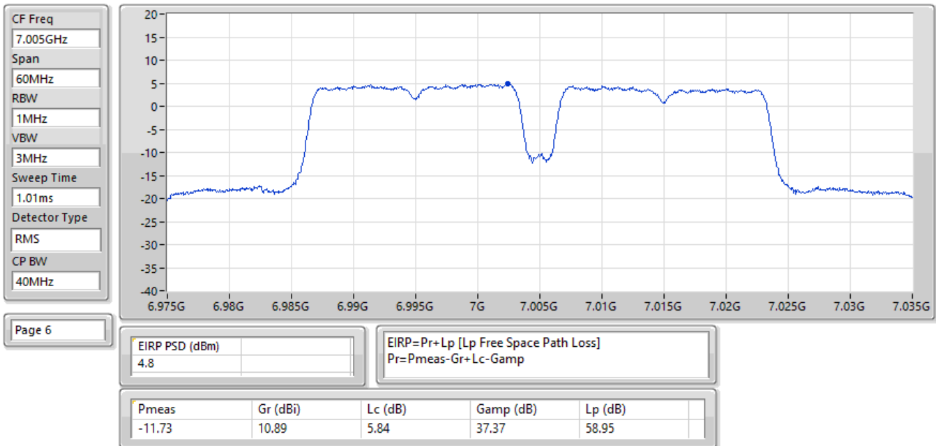
EIRP PSD;Band:7.0G;a40;BWch:40MHz;Nss:1,(6D);Nant:1;Ch:7005MHz;TX
