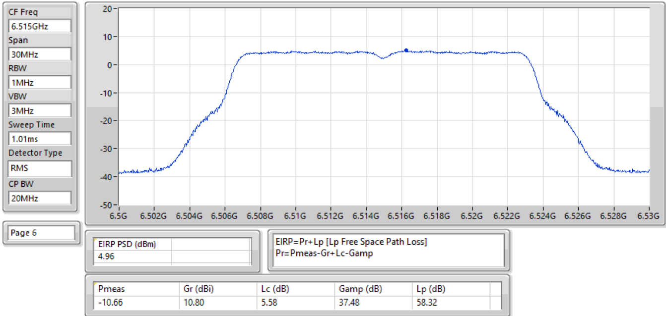
EIRP PSD;Band:6.4G;a20;BWch:20MHz;Nss:1,(6D);Nant:1;Ch:6515MHz;TX
