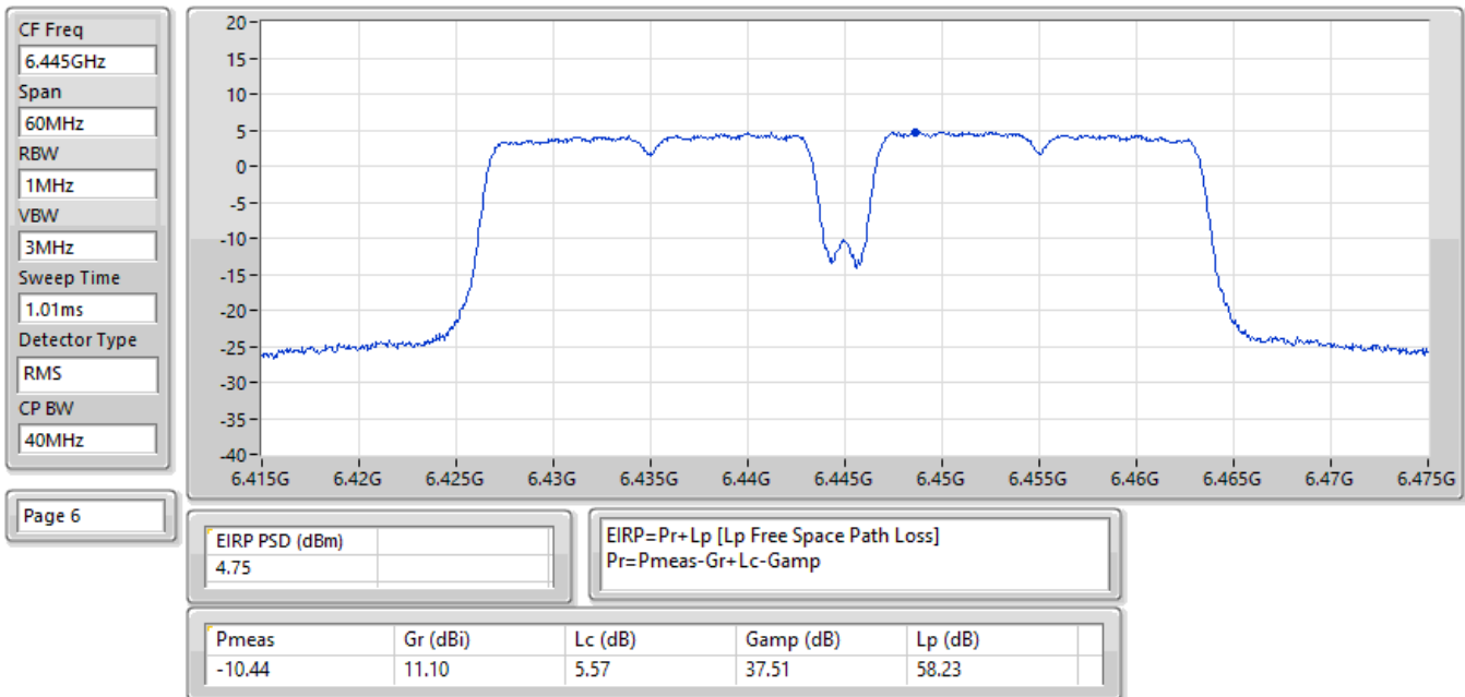
EIRP PSD;Band:6.4G;a40;BWch:40MHz;Nss:1,(6D);Nant:1;Ch:6445MHz;TX
