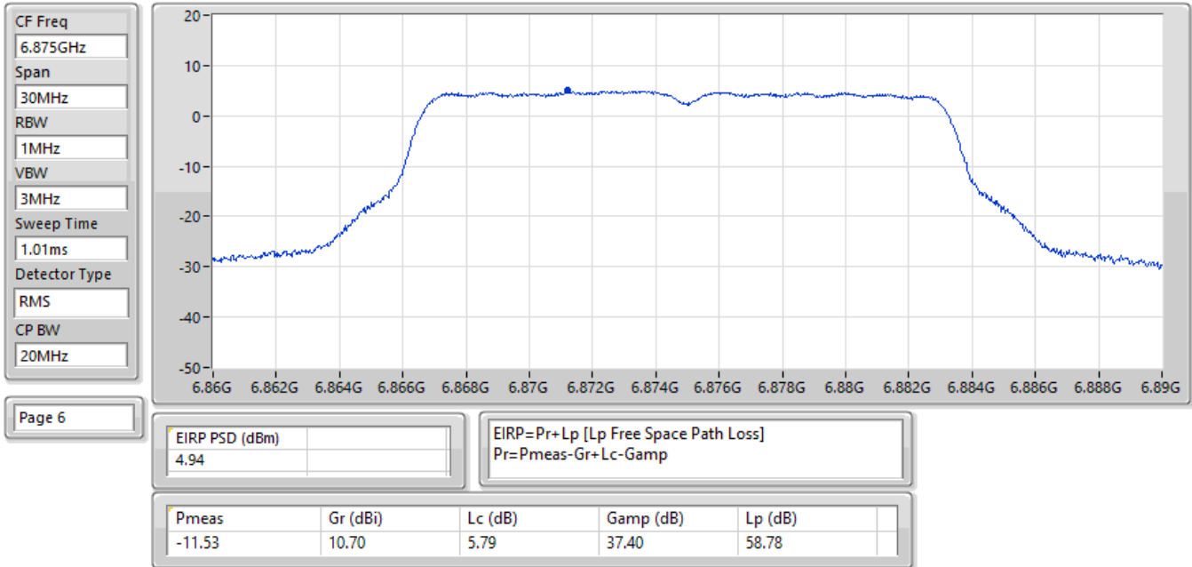
EIRP PSD;Band:6.7G;a20;BWch:20MHz;Nss:1,(6D);Nant:1;Ch:6875MHz;TX
