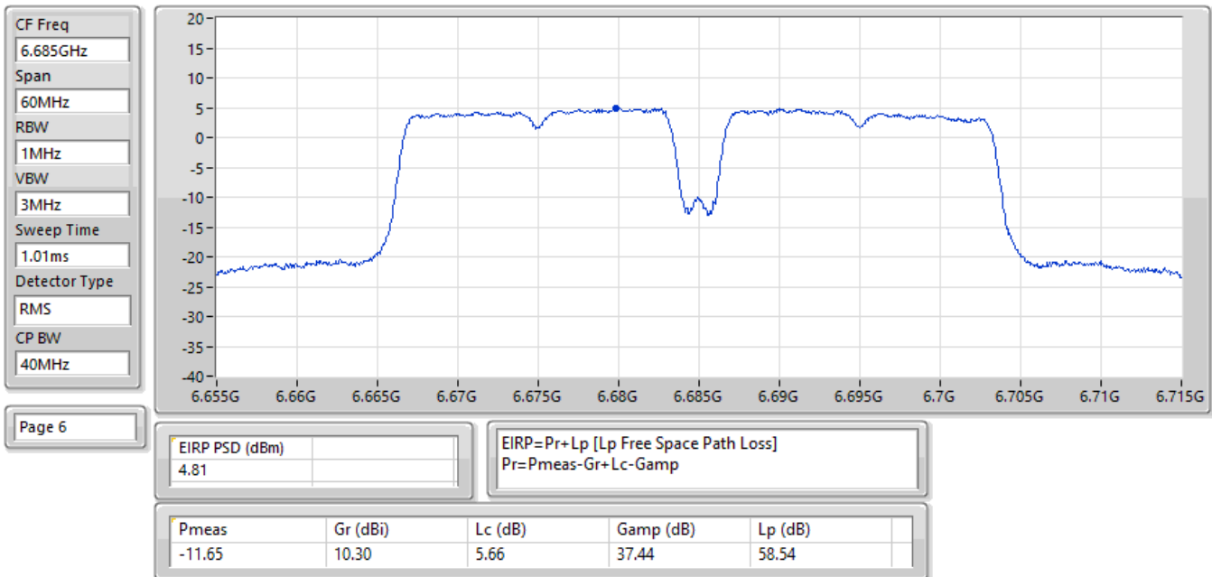
EIRP PSD;Band:6.7G;a40;BWch:40MHz;Nss:1,(6D);Nant:1;Ch:6685MHz;TX
