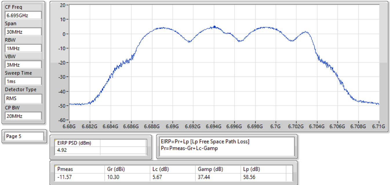
EIRP PSD;Band:6.7G;11a;BWch:20MHz;Nss:1,(6D);Nant:2;Ch:6695MHz;TX
