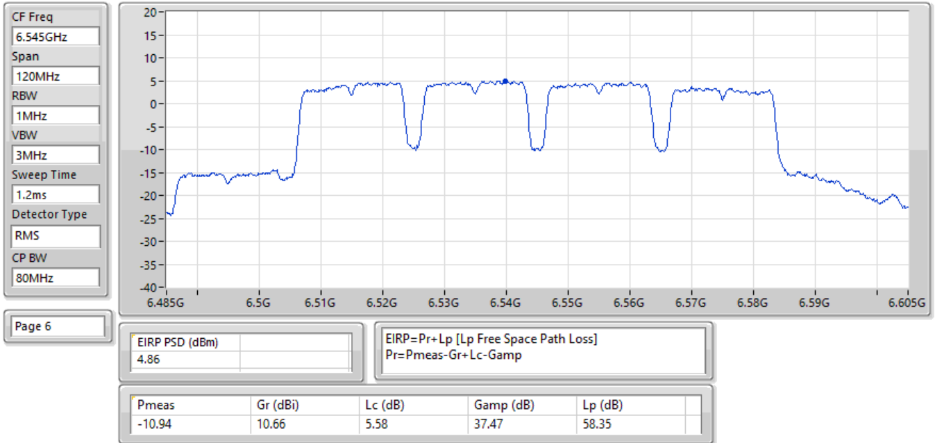
EIRP PSD;Band:6.4G;a80;BWch:80MHz;Nss:1,(6D);Nant:1;Ch:6545MHz;TX
