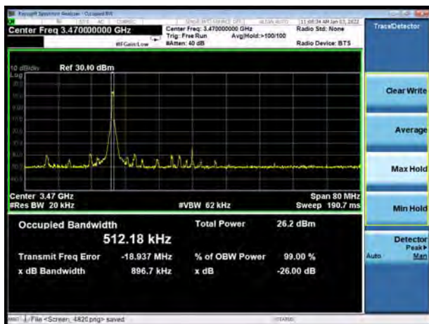
NR n77 Subset 1 QPSK 1RB 40MHz CH-Middle
