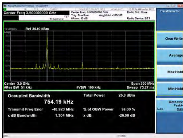
NR n77 Subset 1 QPSK 1RB 100MHz CH-Middle
