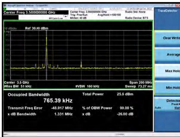
DC_7A-n78 256QAM 1RB 100MHz CH- Middle
