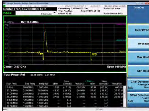
NR n77 Subset 1 40MHz PI/2 BPSK 100%RB CH-Low
