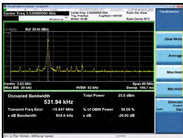
NR n77 Subset 1 QPSK 1RB 40MHz CH-High
