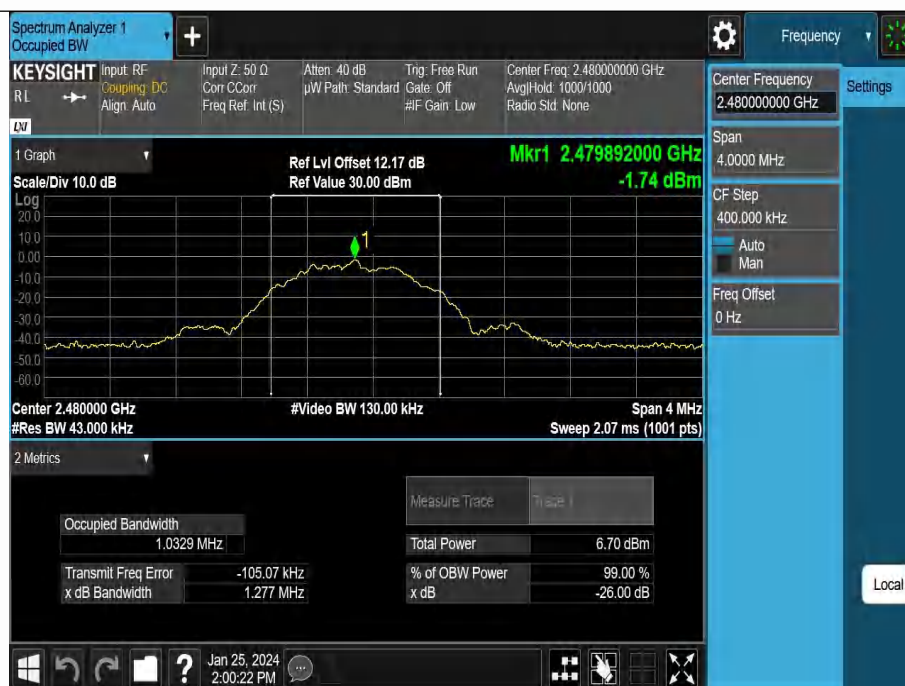
BLE 1M-Ant1-2480
