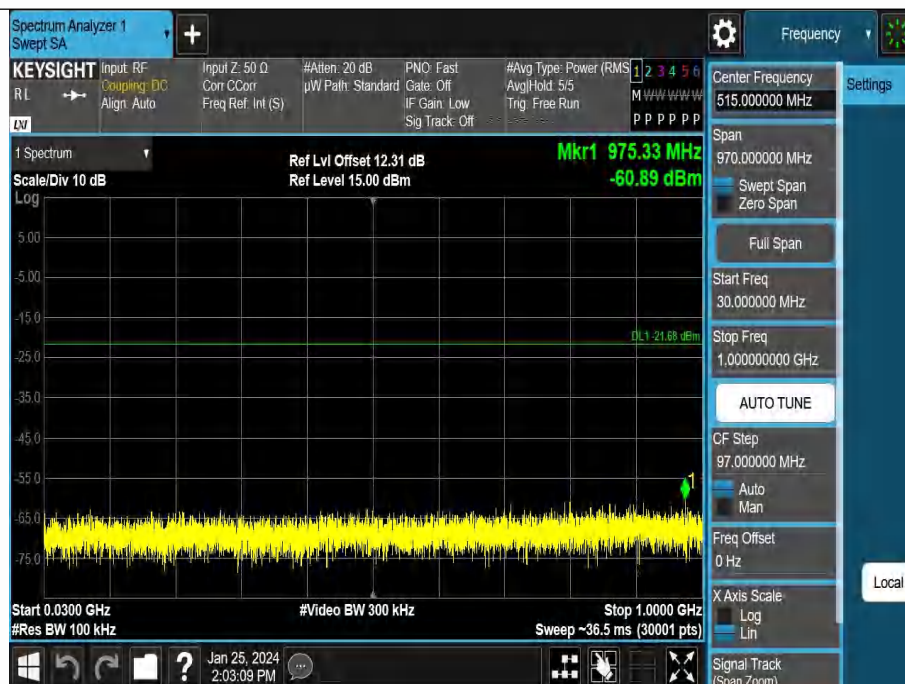
BLE 2M-Ant1-2402-30~1000-PASS
