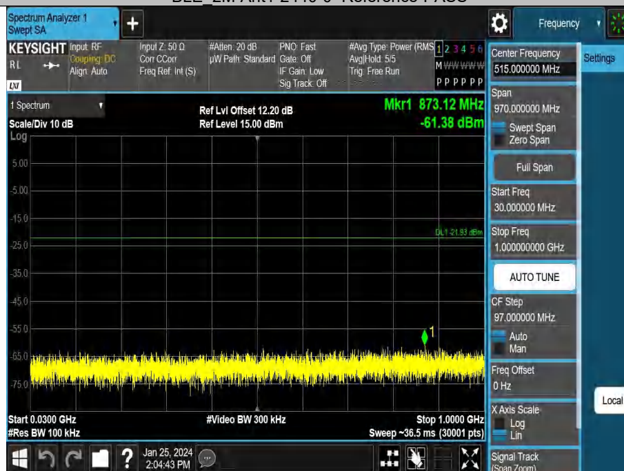
BLE_2M-Ant1-2440-30~1000-PASS
