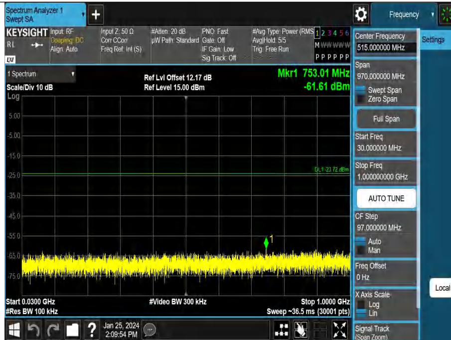
BLE 2M-Ant1-2480-30~1000-PASS
