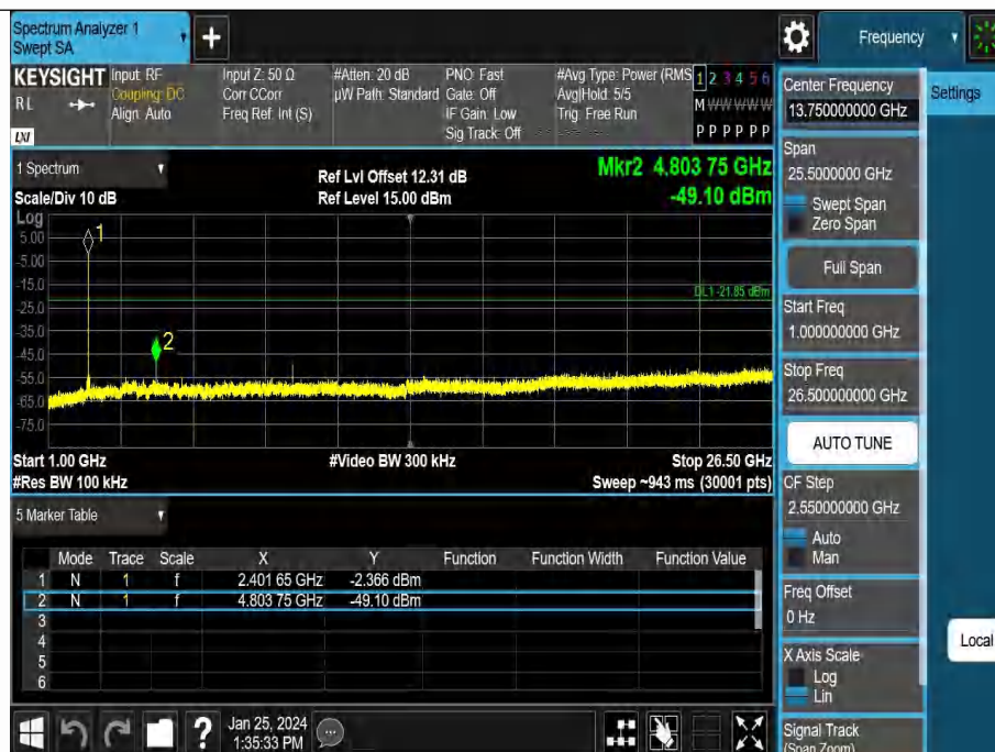
BLE 1M-Ant1-2402-1000~26500-PASS
