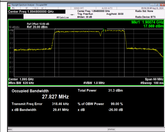
2-2-20MHz-10MHz-QPSK-QPSK-19001-19145-100RB#0-50RB#0-PASS
