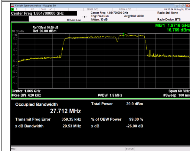
2-2-20MHz-10MHz-16QAM-16QAM-18700-18844-100RB# 0-50RB#0-PASS
