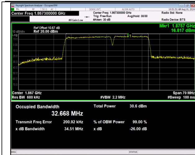
2-2-20MHz-15MHz-QPSK-QPSK-18700-18871-100RB#0-75RB#0-PASS
