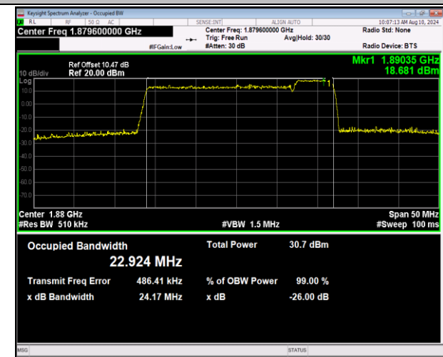
2-2-20MHz-5MHz-QPSK-QPSK-18875-18992-100RB#0-2 5RB#0-PASS
