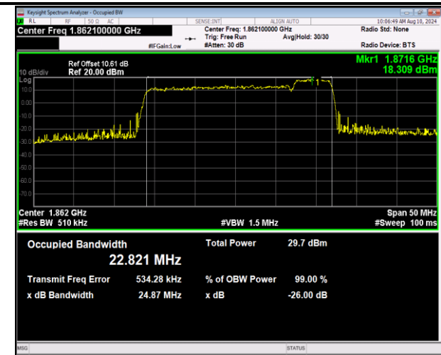
2-2-20MHz-5MHz-16QAM-16QAM-18700-18817-100RB#0-2 -25RB#0-PASS
