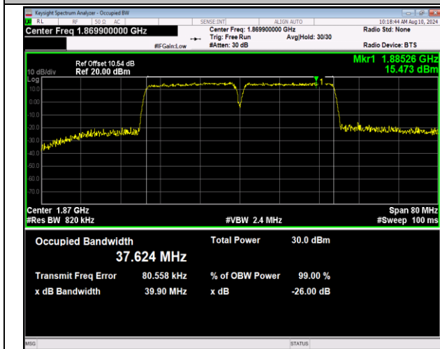
2-2-20MHz-20MHz-16QAM-16QAM-18700-18898-100RB#0-100RB#0-PASS
