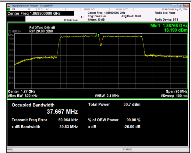
2-2-20MHz-20MHz-QPSK-QPSK-18700-18898-100RB#0-100RB#0-PASS
