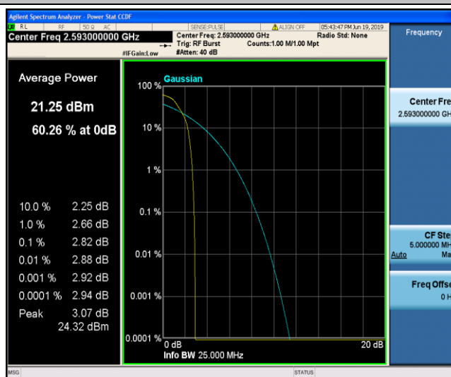
Band41_15MHz_QPSK_40620_1RB#0
