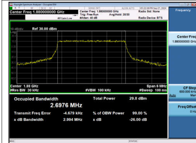
Band2-3MHz-QPSK-18900-15RB#0-PASS
