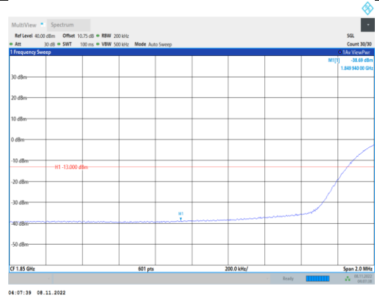
Band2-20MHz-16QAM-18700-100RB#0
