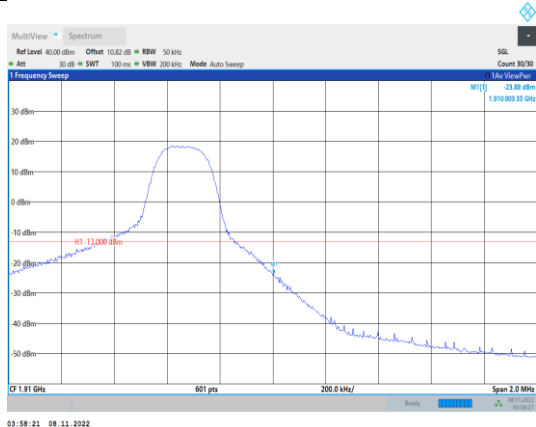
Band2-5MHz-QPSK-19175-1RB#24
