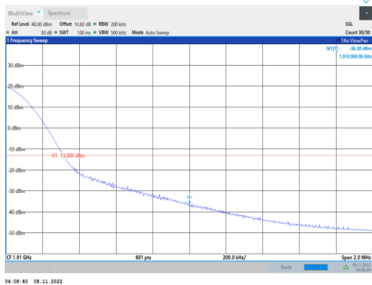
Band2-20MHz-16QAM-19100-1RB#99
