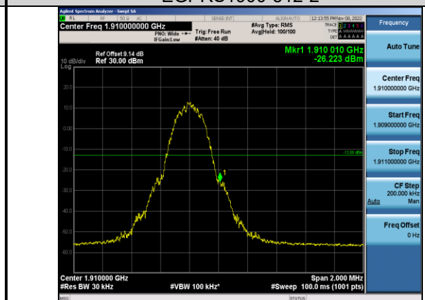
EGPRS1900-810-2
