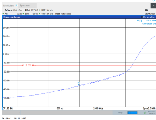
Band2-20MHz-QPSK-18700-1RB#0
