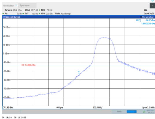
Band2-5MHz-QPSK-18625-1RB#0
