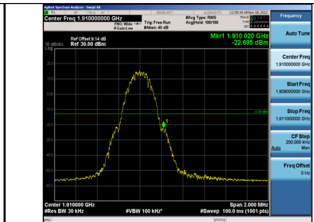
GPRS1900-810-0
