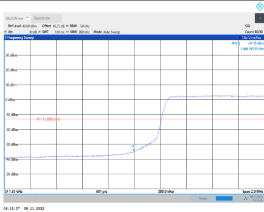
Band2-5MHz-QPSK-18625-25RB#0
