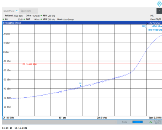
Band2-20MHz-64QAM-18700-1RB#0
