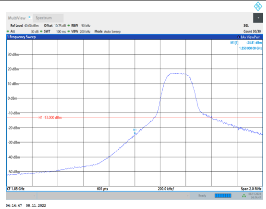
Band2-5MHz-16QAM-18625-1RB#0
