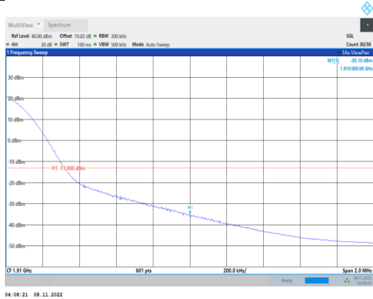
Band2-20MHz-QPSK-19100-1RB#99
