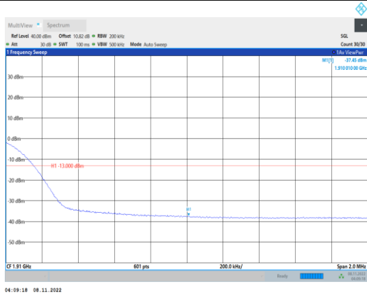
Band2-20MHz-16QAM-19100-100RB#0
