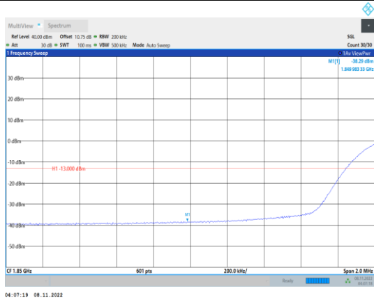
Band2-20MHz-QPSK-18700-100RB#0
