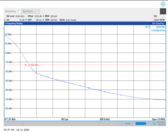
Band2-20MHz-64QAM-19100-1RB#99
