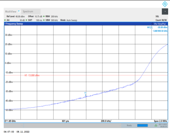
Band2-20MHz-16QAM-18700-1RB#0
