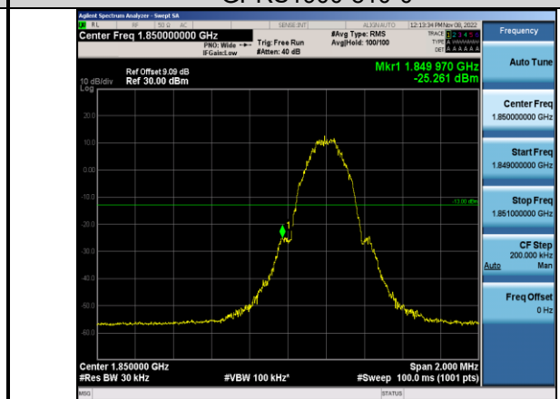
EGPRS1900-512-2
