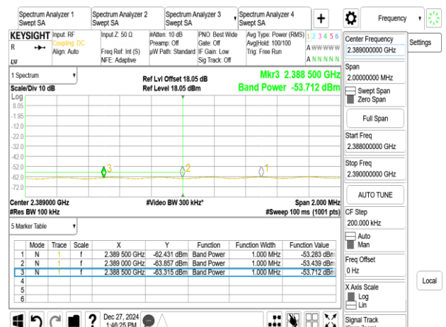
802.11n_40MHz_Chain0_2437MHz_L
