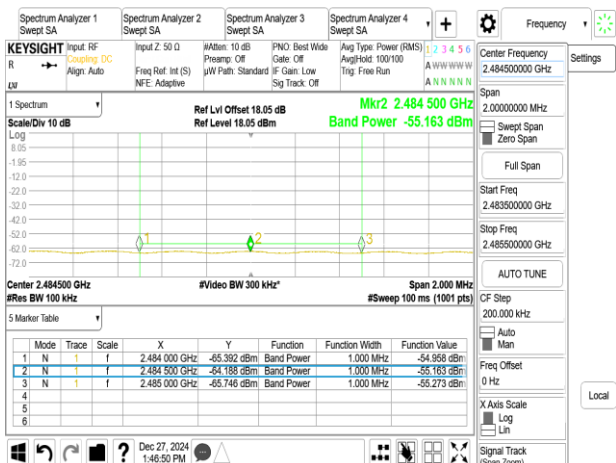
802.11n_40MHz_Chain0_2442MHz
