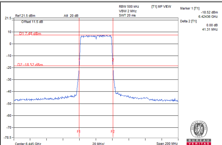
802.11be (EHT40) / Chain 0 : CH 99
