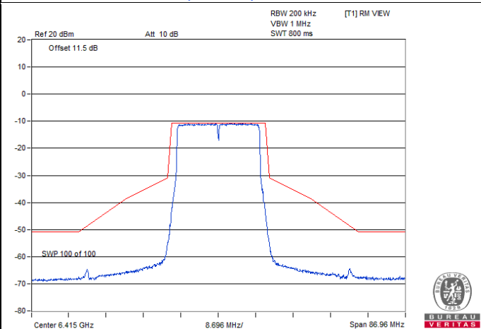
802.11be (EHT20) / Chain 3 : CH 93
