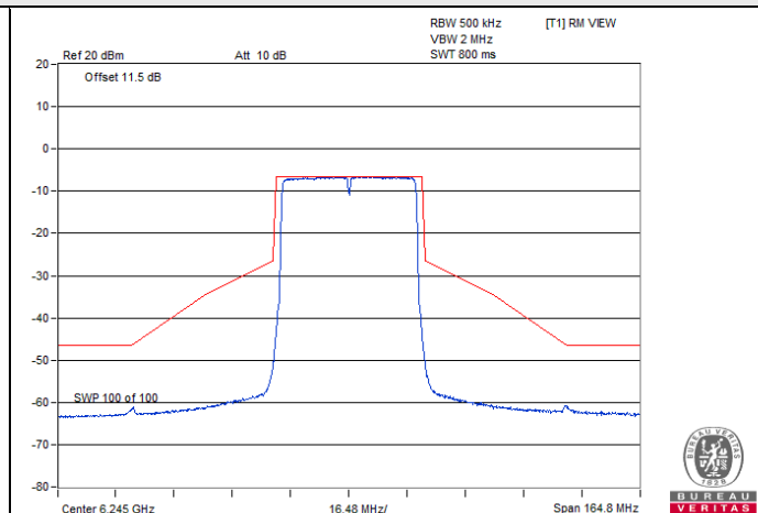
802.11be (EHT40) / Chain 3 : CH 59
