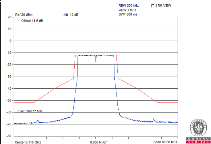
802.11be (EHT20) / Chain 3 : CH 33
