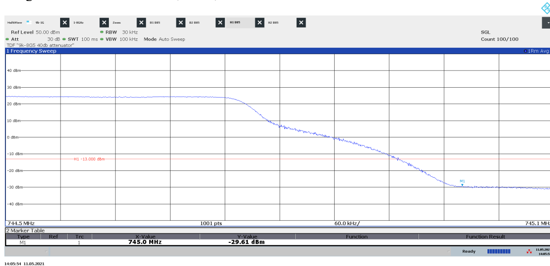
Diagram 2.43a LTE: ETM1.1, T SLTE , Port B:
