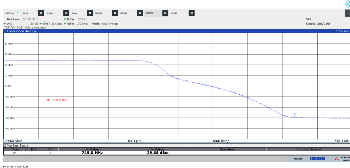
Diagram 2.44a LTE: ETM1.1, T SLTE , Port C:
