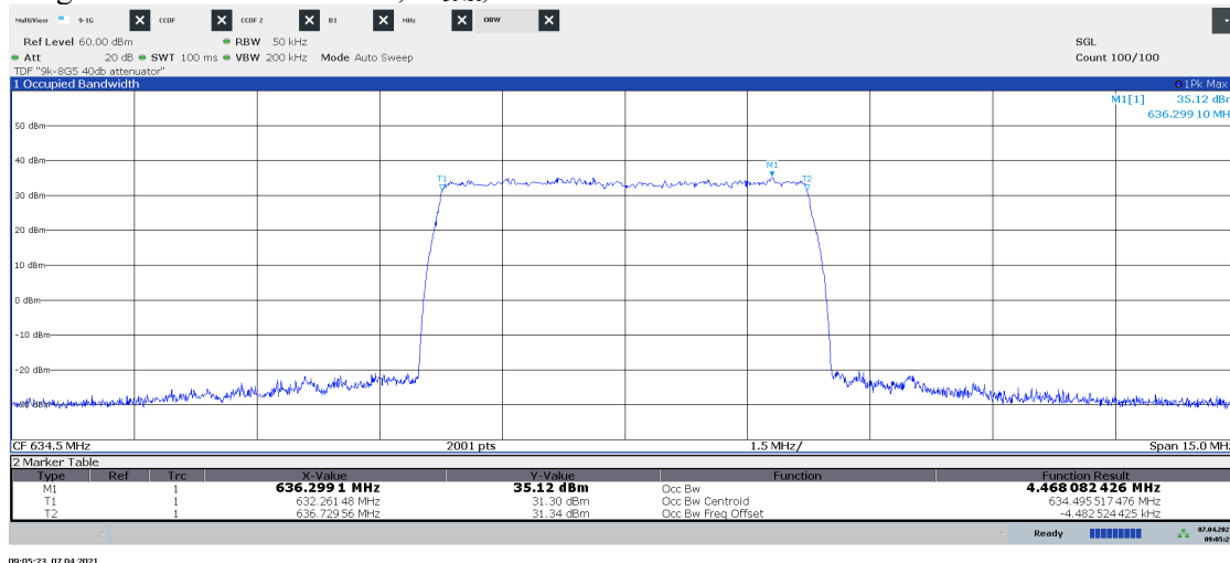
Diagram 1.3 NR: RF1-TM1.1, M 5NR , Port A:
