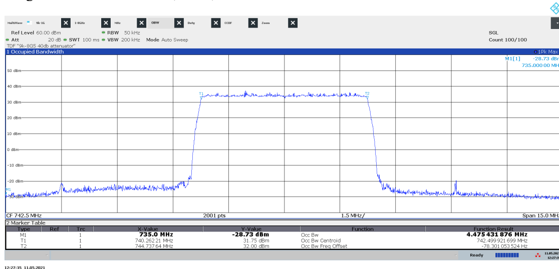
Diagram 1.37 LTE: ETM1.1, T 5LTE , Port A:
