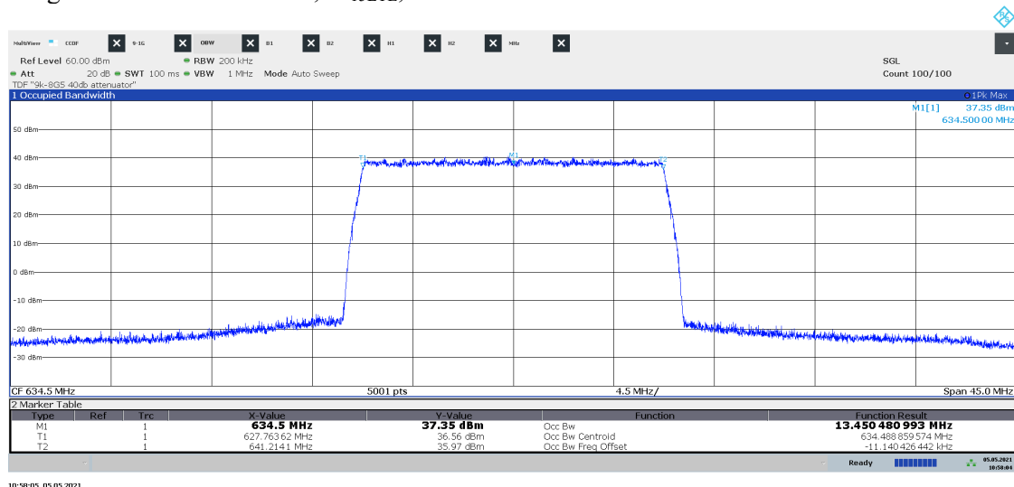
Diagram 1.18 LTE: ETM1.1, M_{15LTE} , Port B:
