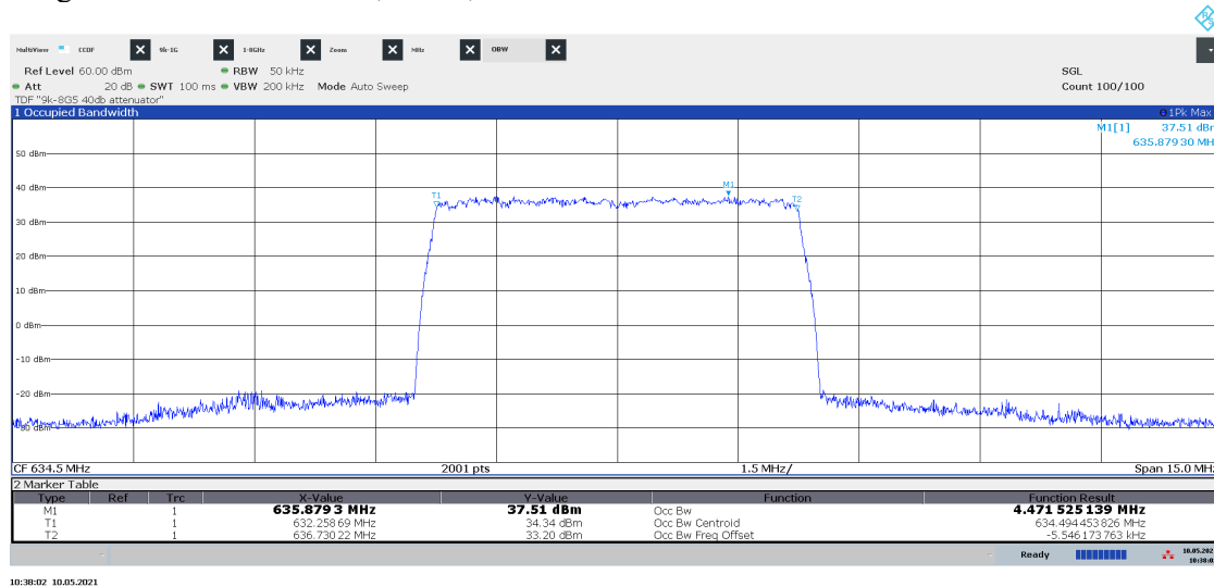
Diagram 1.22 LTE: ETM3.2, M 5LTE , Port B:
