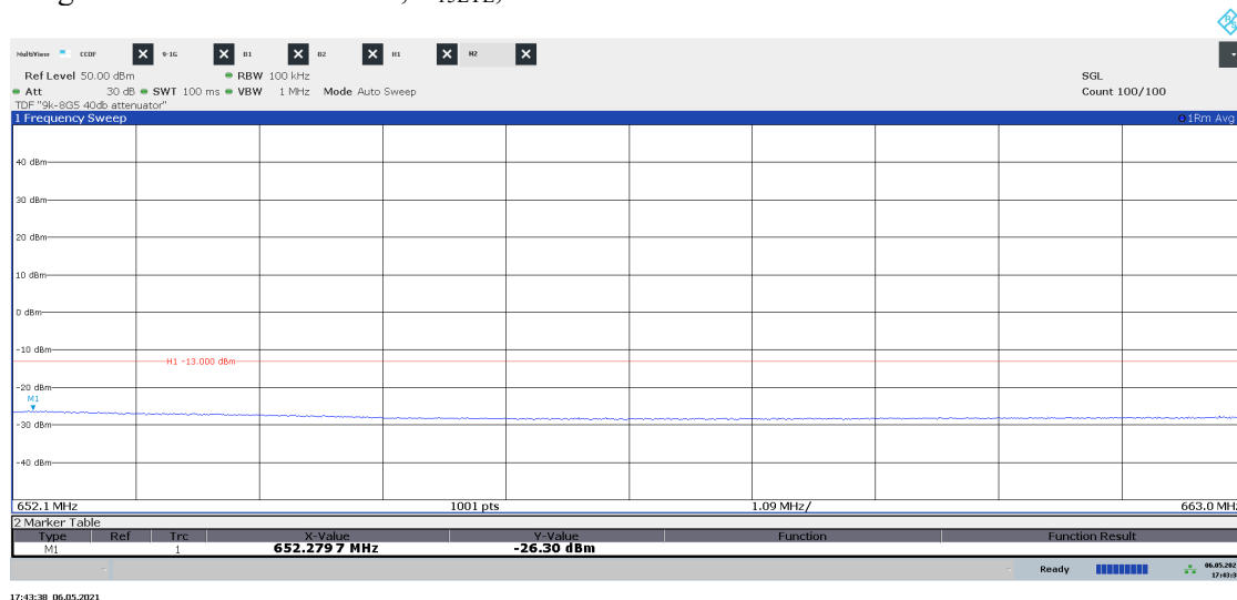
Diagram 2.23b LTE: ETM1.1, T 15LTE , Port B:
