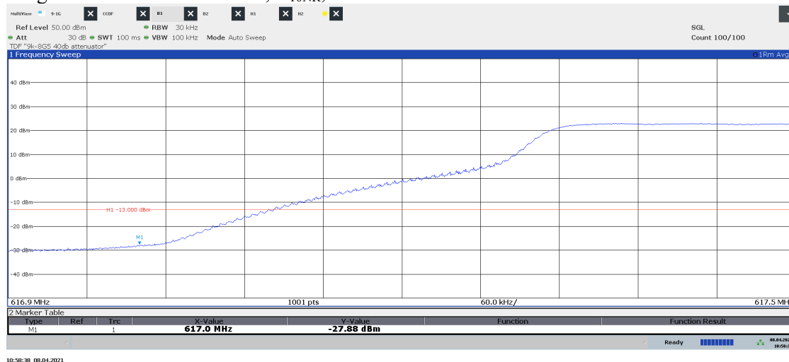
Diagram 2.2a NR: RF1-TM1.1, B 10NR , Port B:
