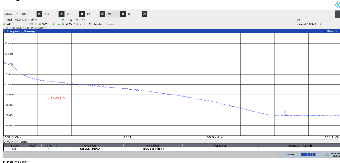
Diagram 2.22a LTE: ETM1.1, T_{10LTE} , Port B:
