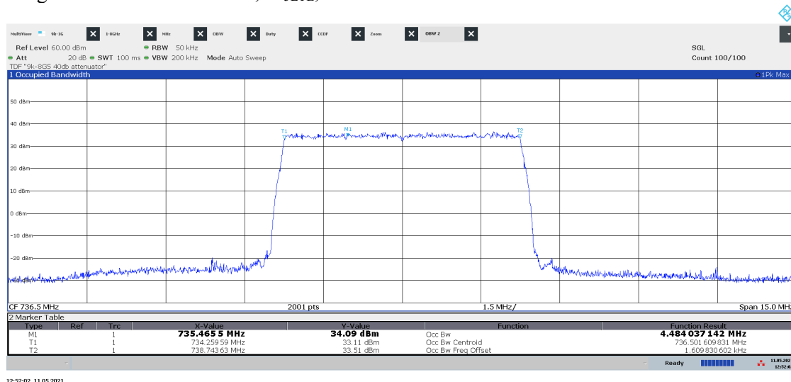
Diagram 1.39 LTE: ETM3.1a, M 5LTE , Port A:
