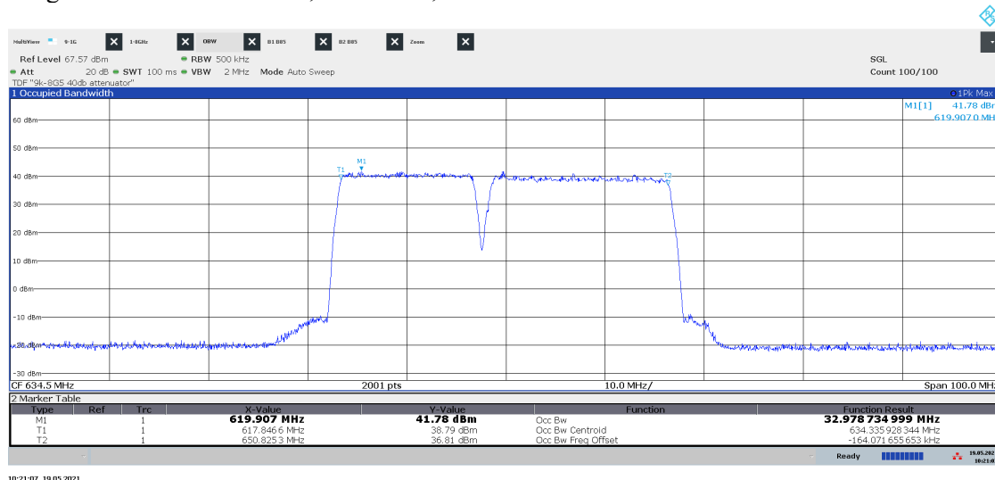
Diagram 1.23 LTE: ETM1.1, CA LTE15+20 , Port B:
