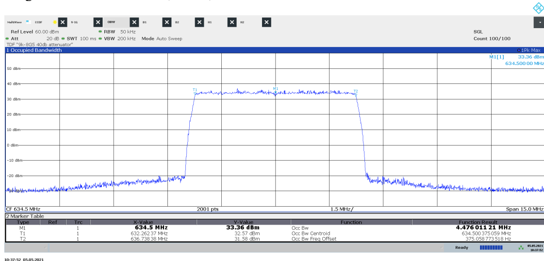
Diagram 1.16 LTE: ETM1.1, M_{5LTE} , Port B:
