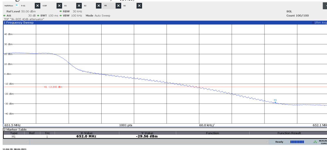
Diagram 2.7a NR: RF1-TM1.1, T 15NR , Port B:
