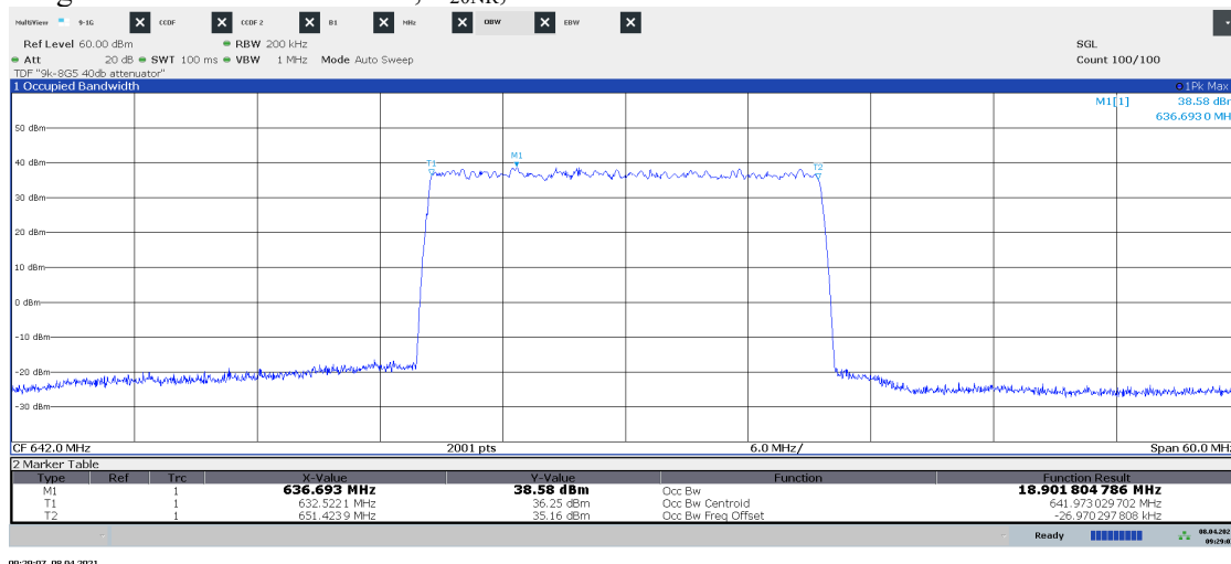
Diagram 1.11 NR: RF1-TM1.1, T 20NR , Port B:
