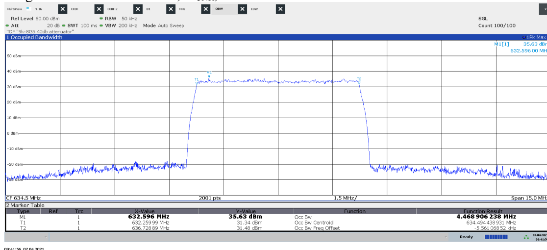
Diagram 1.6 NR: RF1-TM1.1, M 5NR , Port D:
