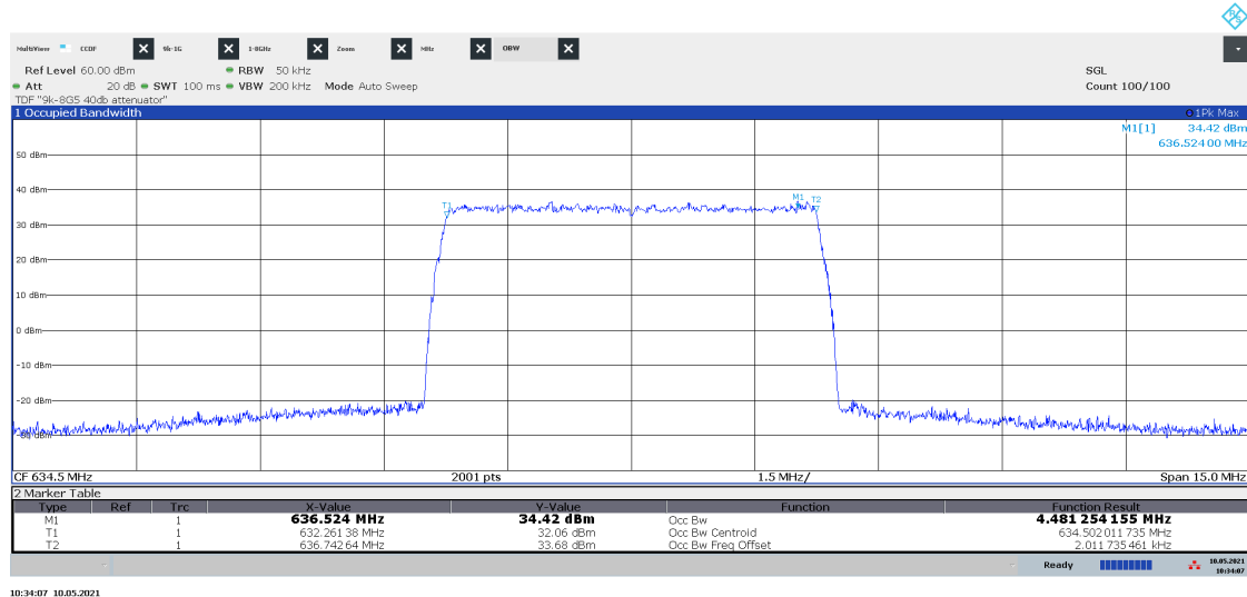
Diagram 1.20 LTE: ETM3.1, M 5LTE , Port B:
