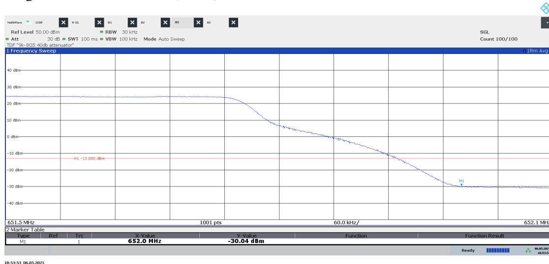
Diagram 2.19a LTE: ETM1.1, T SLTE , Port B:
