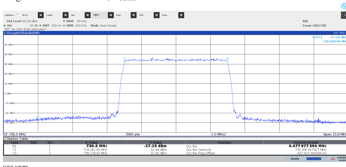
Diagram 1.32 LTE: ETM1.1, M 5LTE , Port A:
