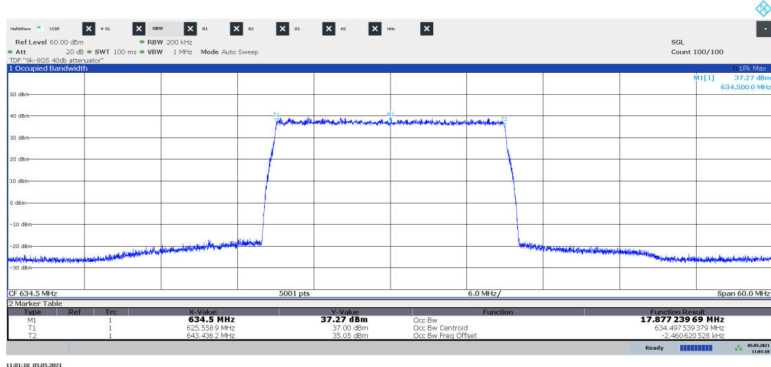
Diagram 1.19 LTE: ETM1.1, M 20LTE , Port B:
