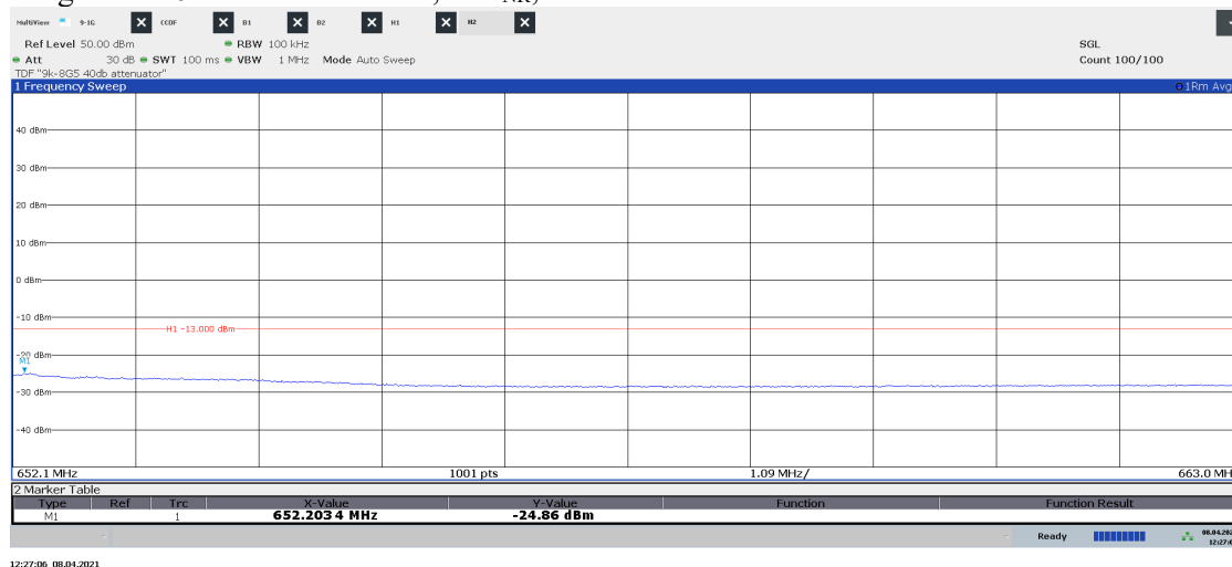
Diagram 2.10b NR: RF1-TM1.1, Tim NR , Port B:
