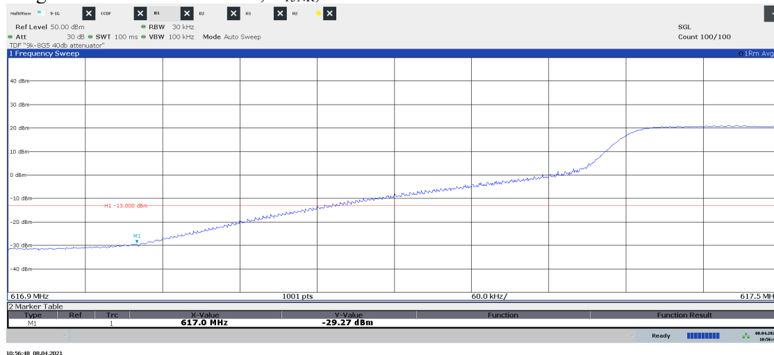
Diagram 2.3a NR: RF1-TM1.1, B 15NR , Port B:
