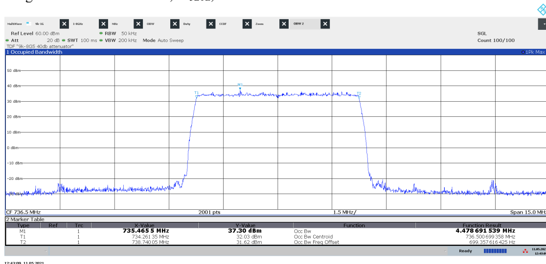
Diagram 1.35 LTE: ETM1.1, M_{5LTE} , Port D:
