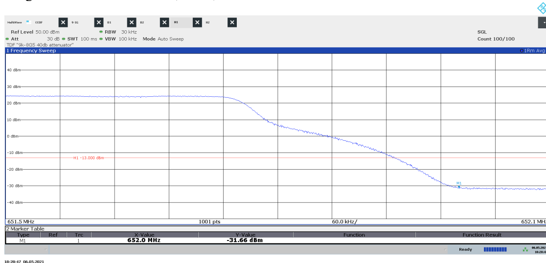
Diagram 2.21a LTE: ETM1.1, T SLTE , Port D:
