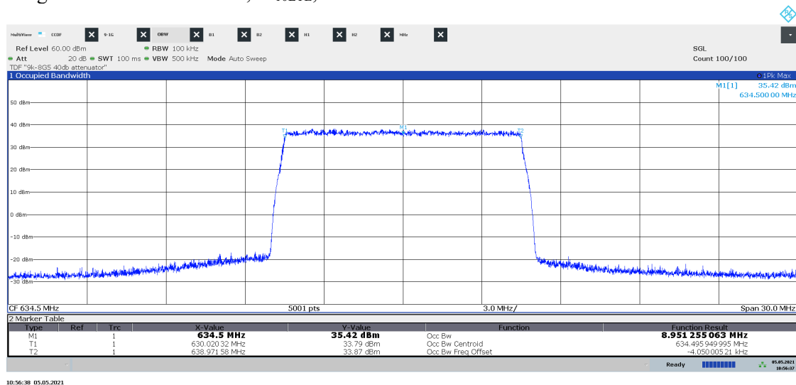
Diagram 1.17 LTE: ETM1.1, M_{10LTE} , Port B:
