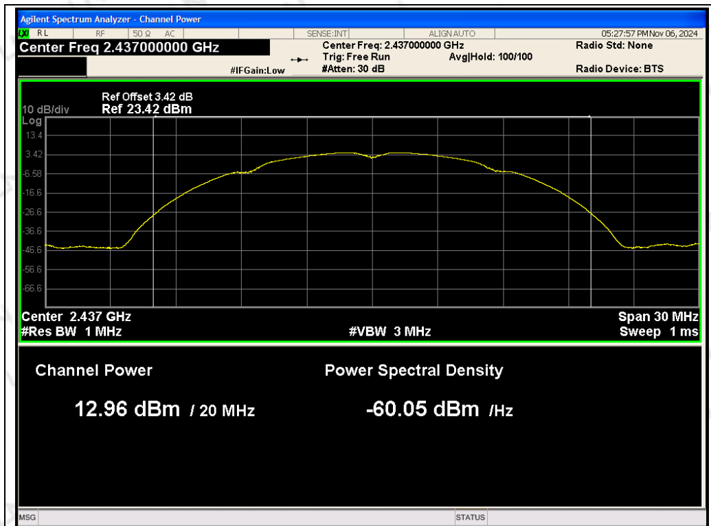
ANT 1 802.11b 2437MHz
