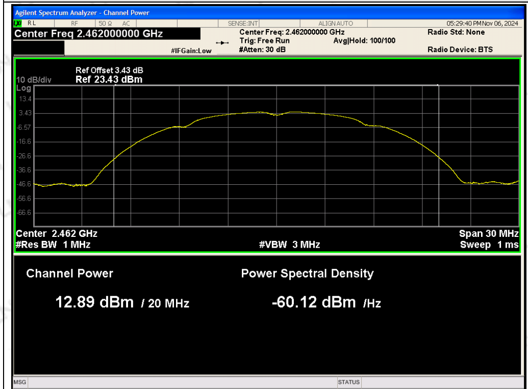
ANT 1 802.11b 2462MHz
