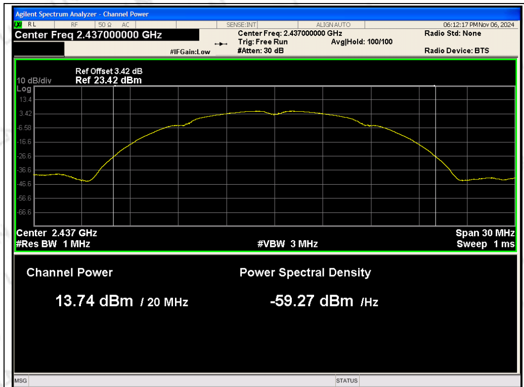
ANT 2 802.11b 2437MHz
