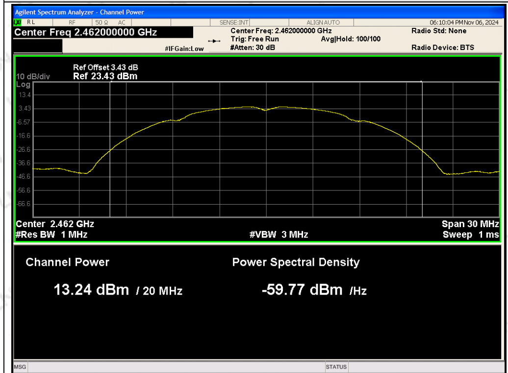
ANT 2 802.11b 2462MHz
