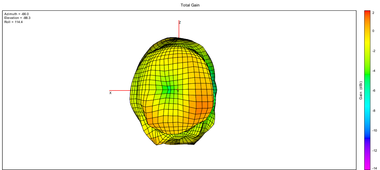
2450MHz_20#_Right
