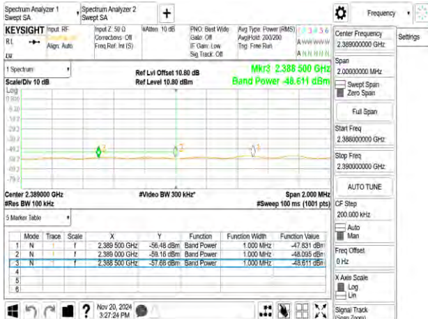
802.11n_20MHz_2422MHz
