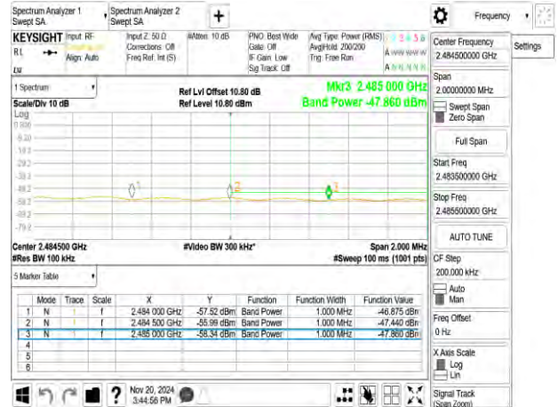
802.11n_20MHz_2457MHz
