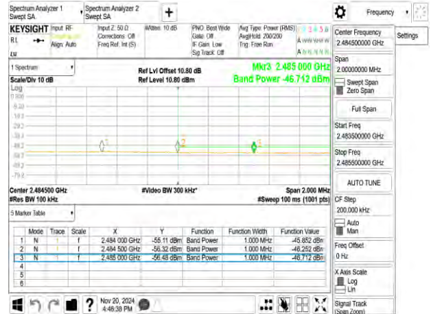
802.11ax_20MHz_2452MHzRU242
