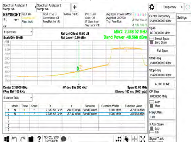
802.11n_20MHz_2422MHz
