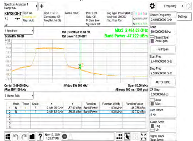
802.11g_20MHz_2472MHz
