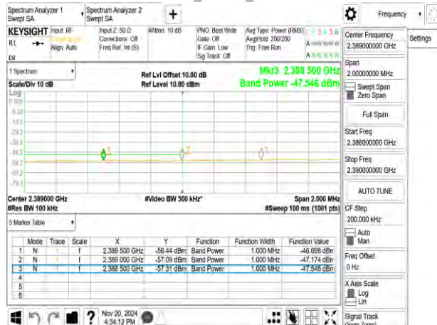
802.11ax_20MHz_2427MHzRU242
