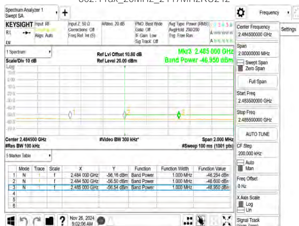
802.11ax_20MHz_2447MHzRU242
