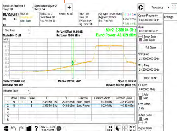
802.11n_20MHz_2417MHz
