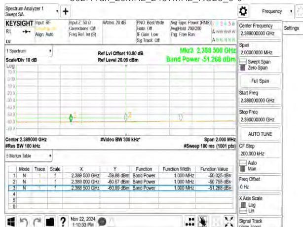
802.11ax_20MHz_2437MHz_RU26_0
