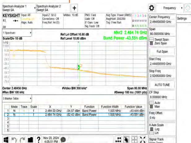
802.11n_40MHz_2452MHz
