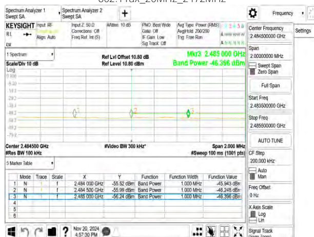
802.11ax_20MHz_2472MHz
