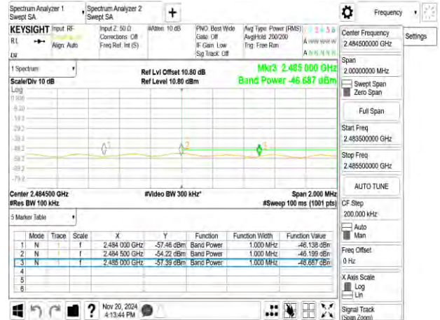
802.11n_40MHz_2457MHz
