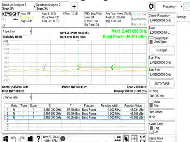
802.11n_40MHz_2447MHz
