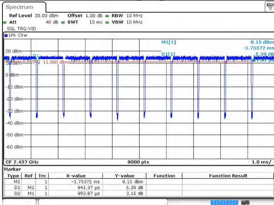
11N40SISO Ant10 2437
