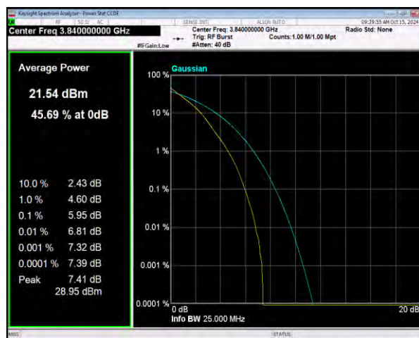
n77(3700-3980) SCS=30kHz DFT_QPSK BW=20MHz Channel=656000 RB=50@0
