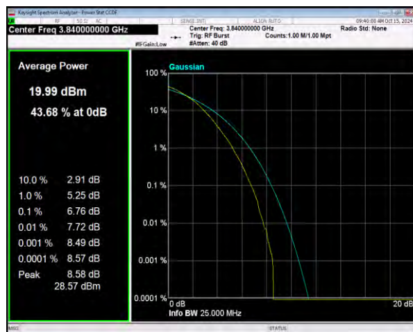
n77(3700-3980) SCS=30kHz DFT_64QAM BW=20MHz Channel=656000 RB=50@0
