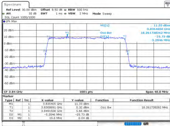
n77(3700-3980) SCS=30kHz CP_16QAM BW=20MHz Channel=656000 RB=51@0
