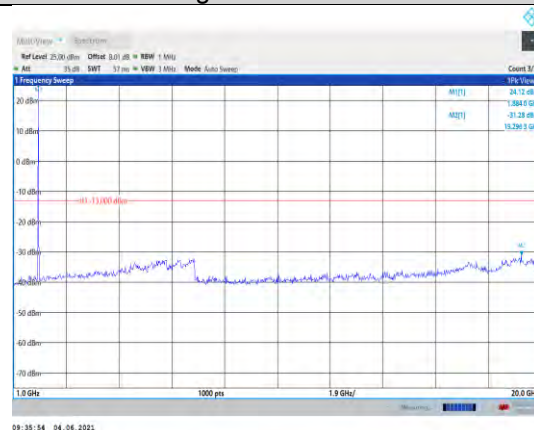
Band25-10MHz-QPSK-26365-1RB#0- Range2:1000~20000MHz
