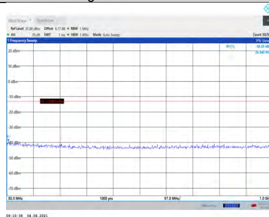
Band4-5MHz-QPSK-20375-1RB#0- Range1:30~1000MHz
