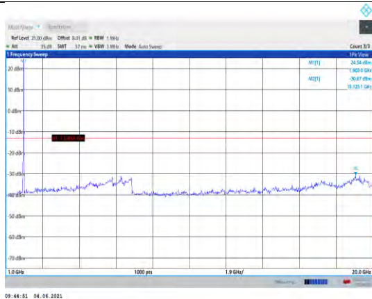
Band25-20MHz-QPSK-26590-1RB#0- Range2:1000~20000MHz
