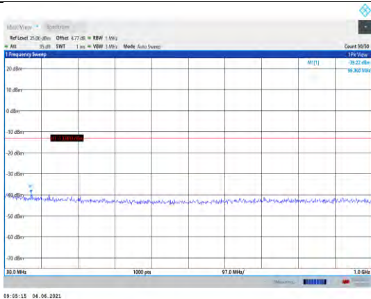
Band4-3MHz-QPSK-19965-1RB#0- Range1:30~1000MHz
