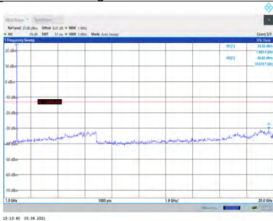
Band2-1.4MHz-QPSK-19193-1RB#0- Range2:1000~20000MHz
