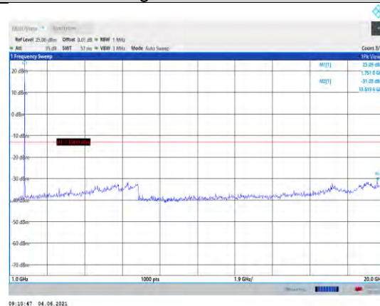
Band4-5MHz-QPSK-20375-1RB#0- Range2:1000~20000MHz
