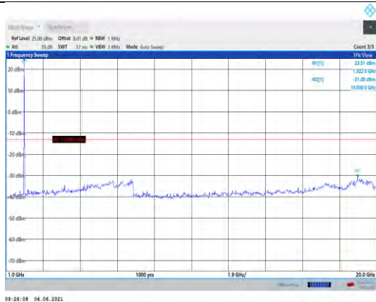
Band25-1.4MHz-QPSK-26683-1RB#0- Range2:1000~20000MHz
