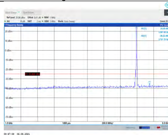
Band41-5MHz-QPSK-40620-1RB#0- Range2:1000~3000MHz
