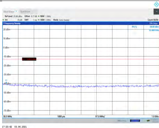
Band2-20MHz-QPSK-18700-1RB#0- Range1:30~1000MHz
