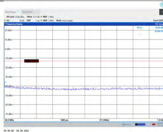
Band25-10MHz-QPSK-26365-1RB#0- Range1:30~1000MHz
