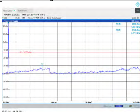
Band2-20MHz-QPSK-18700-1RB#0- Range2:1000~20000MHz
