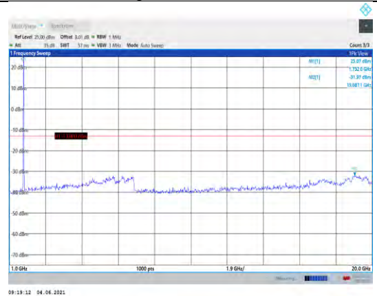
Band4-15MHz-QPSK-20325-1RB#0- Range2:1000~20000MHz
