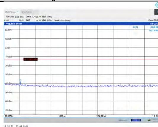
Band2-5MHz-QPSK-19175-1RB#0- Range1:30~1000MHz
