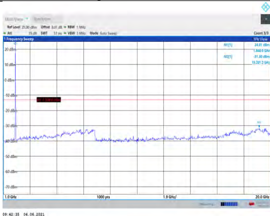
Band25-20MHz-QPSK-26140-1RB#0- Range2:1000~20000MHz
