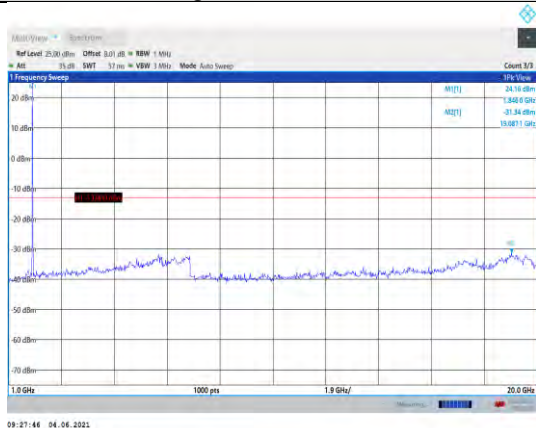
Band25-3MHz-QPSK-26055-1RB#0- Range2:1000~20000MHz
