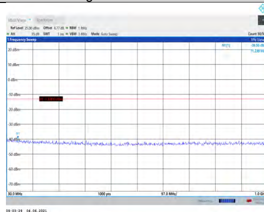
Band4-1.4MHz-QPSK-20393-1RB#0- Range1:30~1000MHz
