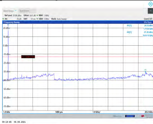
Band4-15MHz-QPSK-20025-1RB#0- Range2:1000~20000MHz
