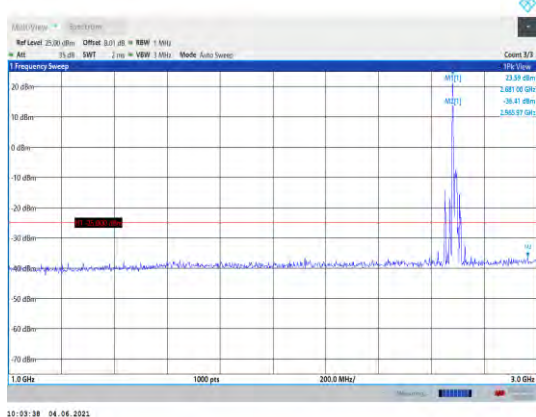
Band41-10MHz-QPSK-41540-1RB#0- Range2:1000~3000MHz
