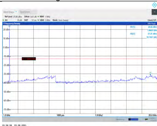
Band2-5MHz-QPSK-18625-1RB#0- Range2:1000~20000MHz
