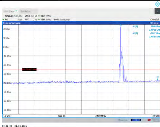
Band41-10MHz-QPSK-39700-1RB#0-Range2:1000~3000MHz
