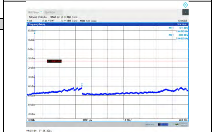
Band2-9538-1000~20000MHz
