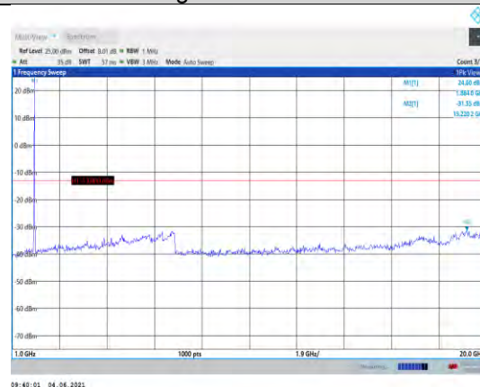
Band25-15MHz-QPSK-26365-1RB#0- Range2:1000~20000MHz
