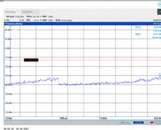
Band4-20MHz-QPSK-20175-1RB#0- Range2:1000~20000MHz
