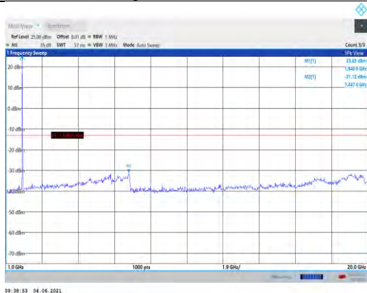
Band25-15MHz-QPSK-26115-1RB#0- Range2:1000~20000MHz
