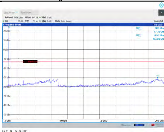
Band4-1.4MHz-QPSK-19957-1RB#0- Range2:1000~20000MHz
