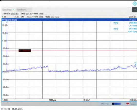
Band4-3MHz-QPSK-19965-1RB#0- Range2:1000~20000MHz
