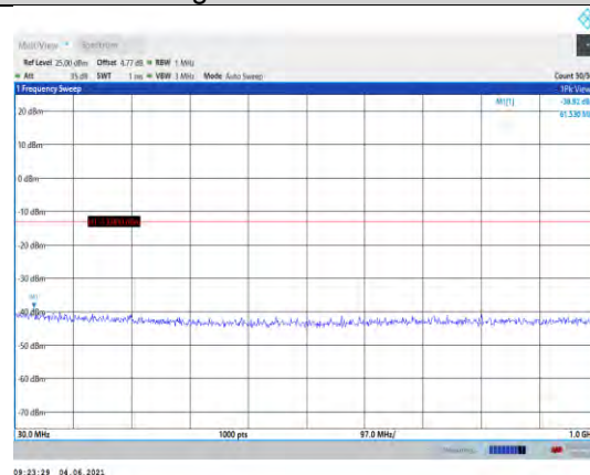
Band4-20MHz-QPSK-20300-1RB#0- Range1:30~1000MHz
