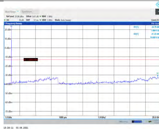
Band2-3MHz-QPSK-18900-1RB#0-Range2:1000~20000MHz
