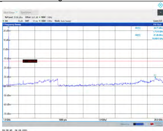
Band4-5MHz-QPSK-19975-1RB#0- Range2:1000~20000MHz
