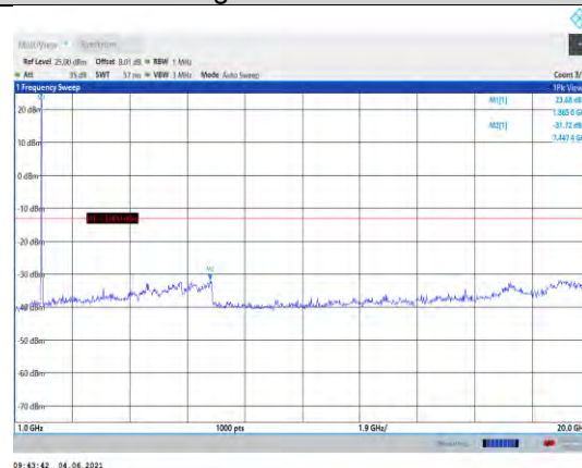
Band25-20MHz-QPSK-26365-1RB#0- Range2:1000~20000MHz
