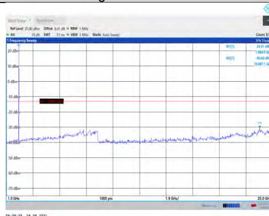
Band25-3MHz-QPSK-26365-1RB#0- Range2:1000~20000MHz
