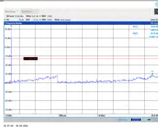
Band2-5MHz-QPSK-18900-1RB#0- Range2:1000~20000MHz
