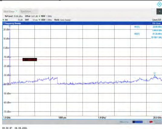
Band25-5MHz-QPSK-26065-1RB#0- Range2:1000~20000MHz
