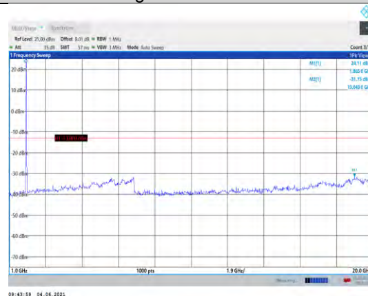
Band25-20MHz-16QAM-26365-1RB#0- Range2:1000~20000MHz
