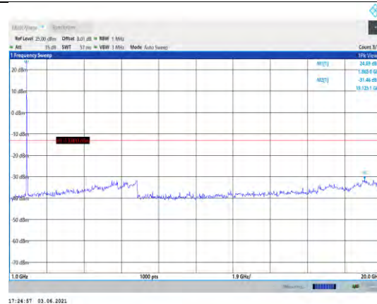
Band2-20MHz-QPSK-18900-1RB#0- Range2:1000~20000MHz
