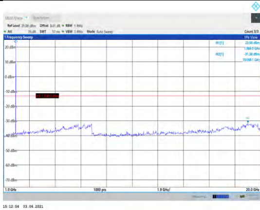
Band2-1.4MHz-QPSK-18900-1RB#0- Range2:1000~20000MHz
