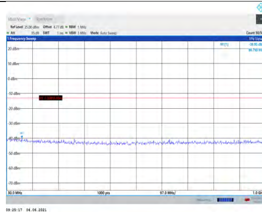
Band25-1.4MHz-QPSK-26365-1RB#0- Range1:30~1000MHz
