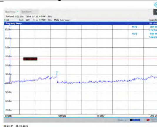
Band4-20MHz-QPSK-20300-1RB#0- Range2:1000~20000MHz
