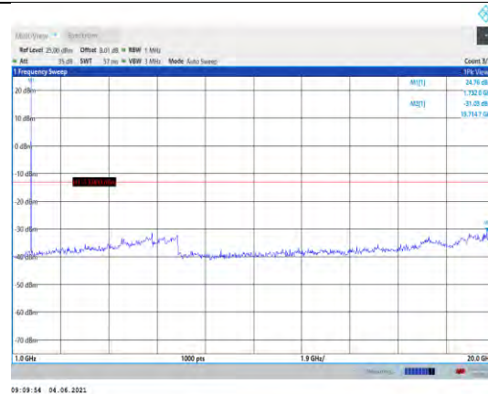
Band4-5MHz-QPSK-20175-1RB#0- Range2:1000~20000MHz
