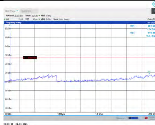
Band4-1.4MHz-QPSK-20393-1RB#0- Range2:1000~20000MHz
