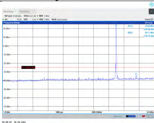
Band41-5MHz-QPSK-39675-1RB#0- Range2:1000~3000MHz
