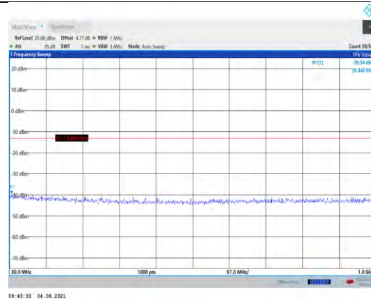
Band25-20MHz-QPSK-26365-1RB#0- Range1:30~1000MHz
