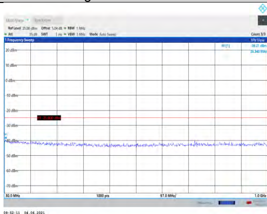
Band41-10MHz-QPSK-39700-1RB#0-Range1:30~1000MHz
