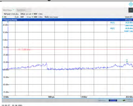
Band2-3MHz-QPSK-18615-1RB#0-Range2:1000~20000MHz
