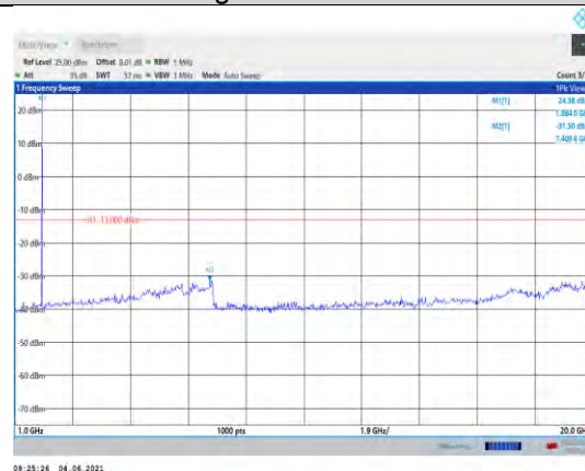
Band25-1.4MHz-QPSK-26365-1RB#0- Range2:1000~20000MHz
