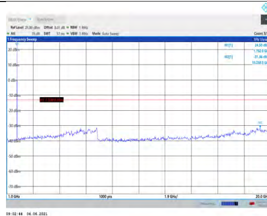
Band4-1.4MHz-QPSK-20175-1RB#0- Range2:1000~20000MHz
