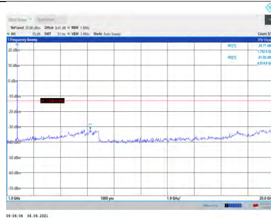
Band4-3MHz-QPSK-20175-1RB#0- Range2:1000~20000MHz
