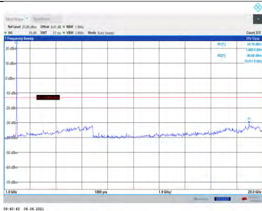
Band25-15MHz-QPSK-26615-1RB#0- Range2:1000~20000MHz
