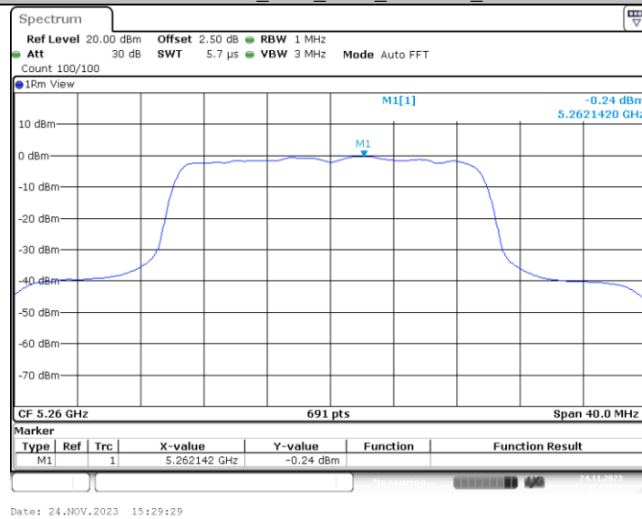
11AX20MIMO_Ant2_5260_242Tone_RU61
