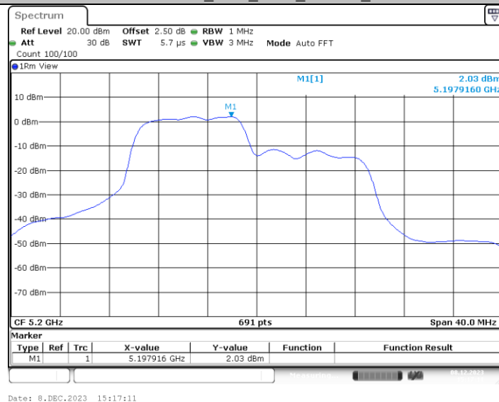
11AX20MIMO_Ant3_5200_106Tone_RU53
