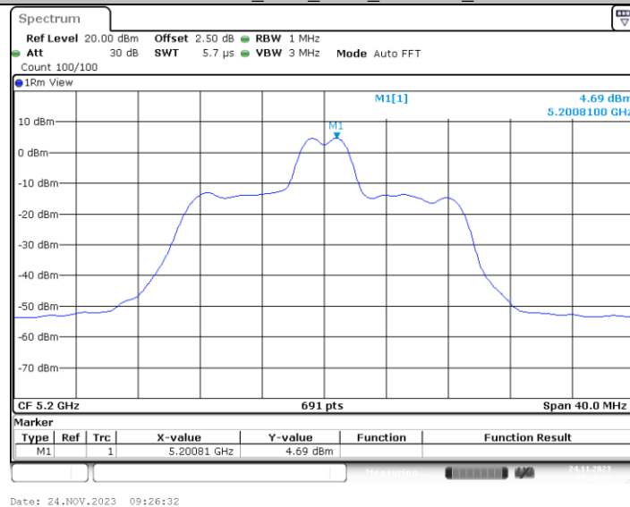
11AX20MIMO_Ant1_5200_26Tone_RU4
