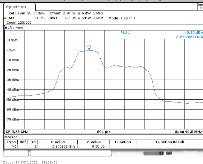
11AX20MIMO_Ant1_5280_52Tone_RU38
