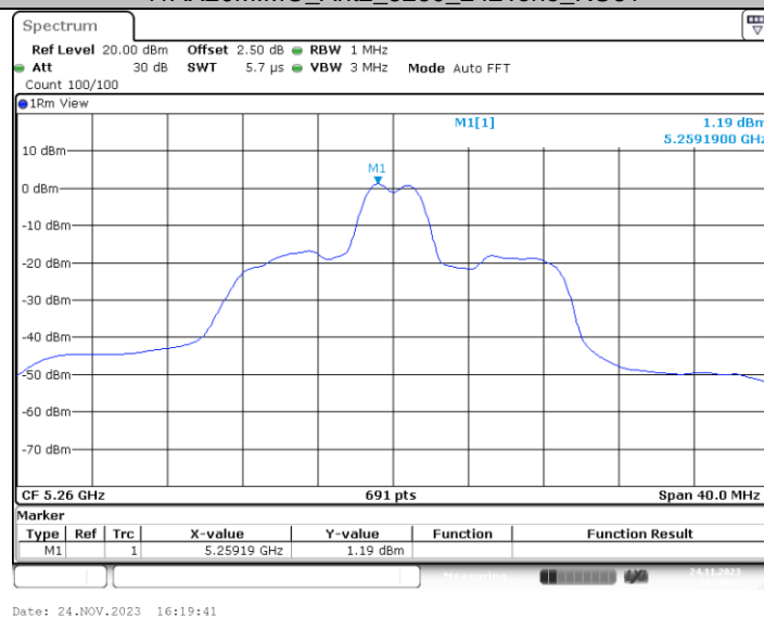
11AX20MIMO_Ant3_5260_26Tone_RU4
