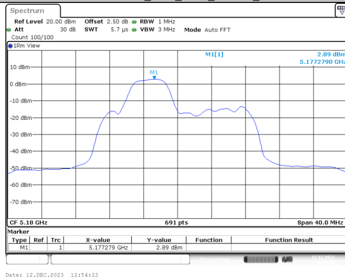
11AX20MIMO_Ant1_5180_52Tone_RU38
