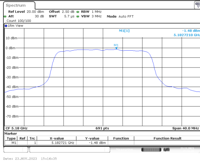
11AX20MIMO_Ant4_5180_242Tone_RU61
