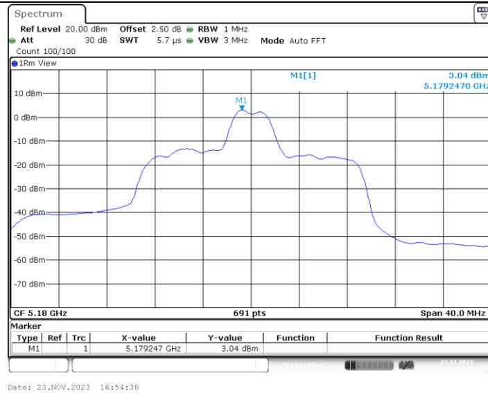
11AX20MIMO_Ant1_5180_26Tone_RU4
