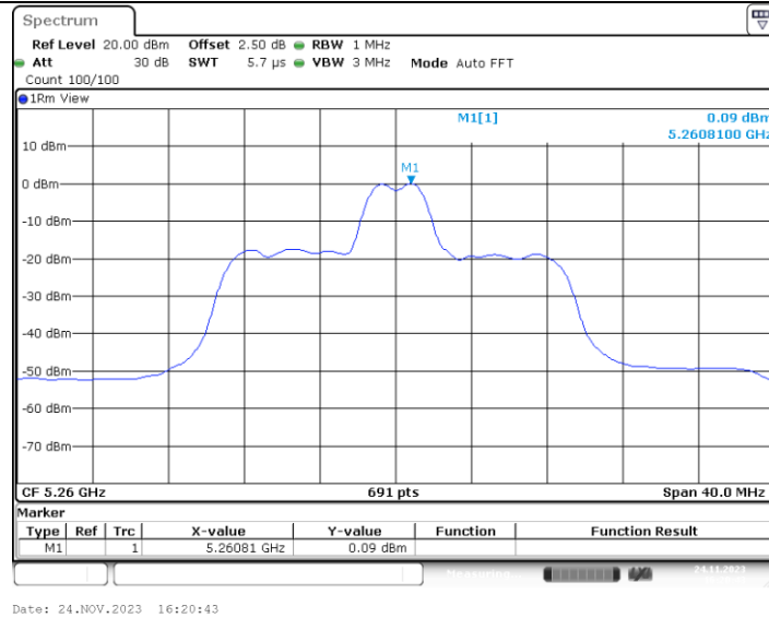
11AX20MIMO_Ant4_5260_26Tone_RU4
