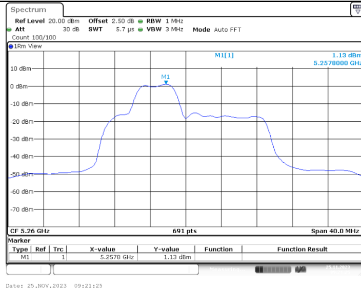
11AX20MIMO_Ant1_5260_52Tone_RU38
