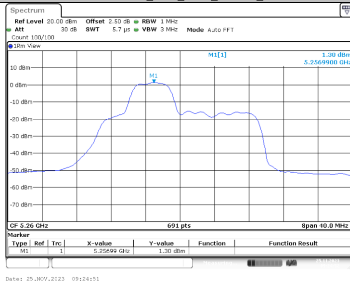
11AX20MIMO_Ant4_5260_52Tone_RU38
