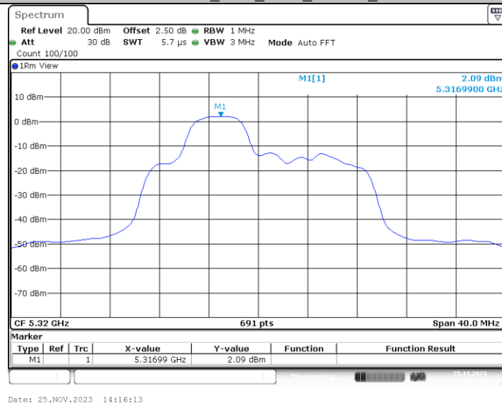
11AX20MIMO_Ant2_5320_52Tone_RU38
