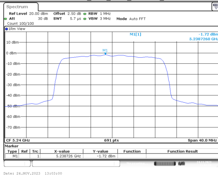
11AX20MIMO_Ant1_5240_242Tone_RU61
