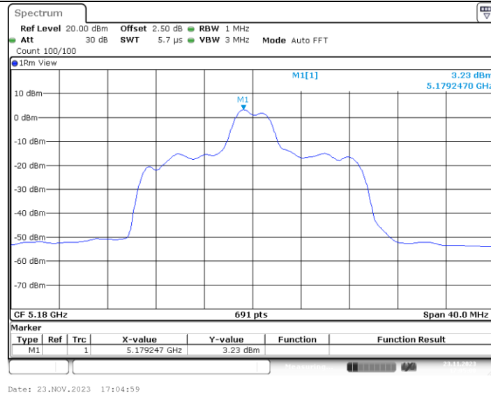
11AX20MIMO_Ant4_5180_26Tone_RU4
