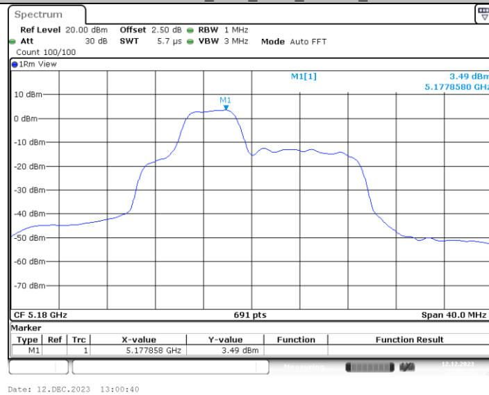
11AX20MIMO_Ant4_5180_52Tone_RU38
