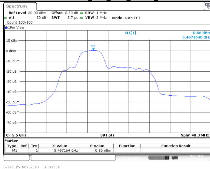
11AX20MIMO_Ant1_5500_52Tone_RU38
