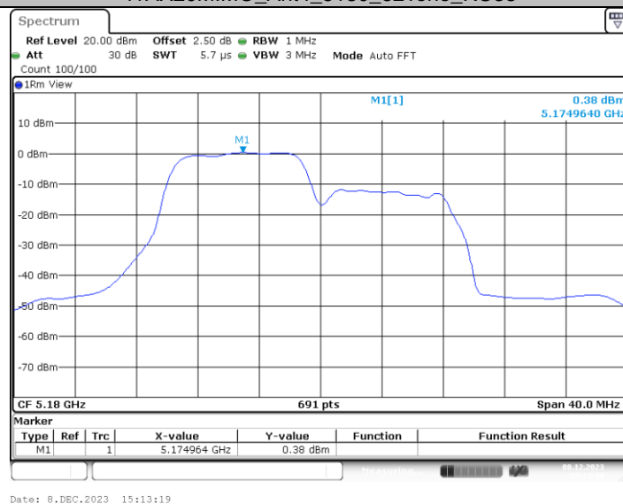
11AX20MIMO_Ant4_5180_106Tone_RU53
