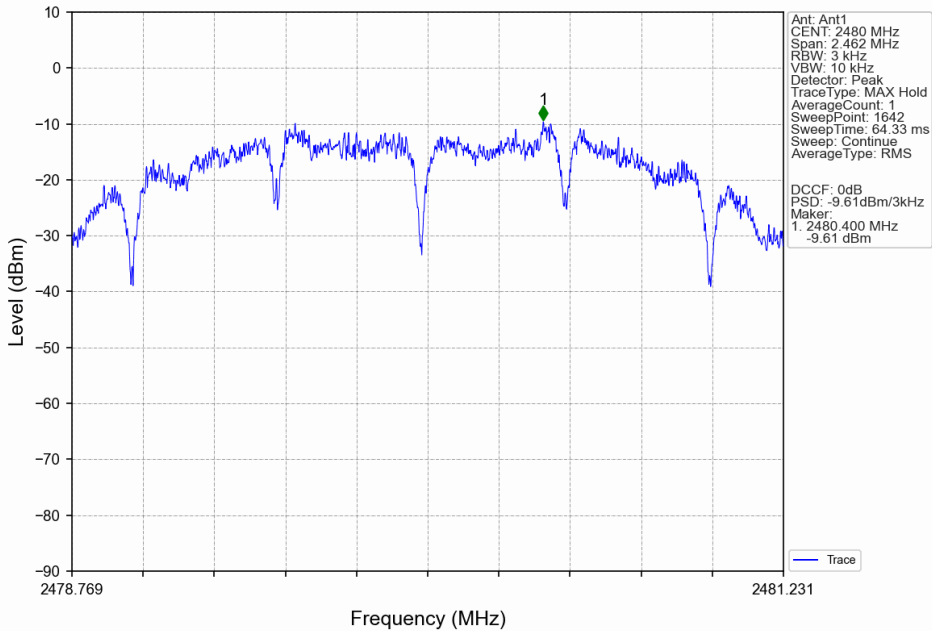
Zigbee_HCH_2480MHz_Ant1_NTNV
